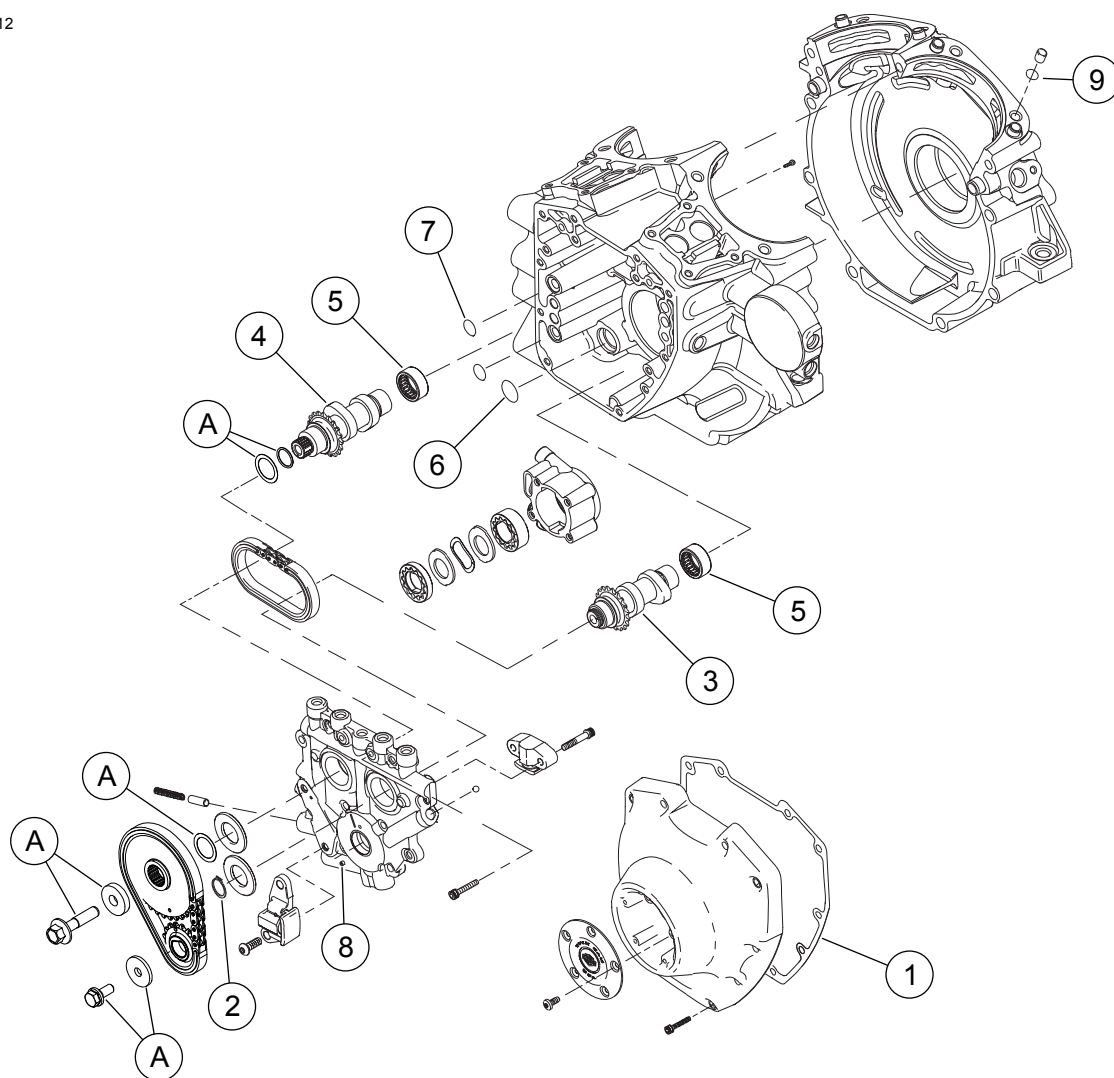
Slika 3. Servisni deli: Dirkalni komplet Screamin' Eagle Twin Cam 110 (1800 cc) Stage V
