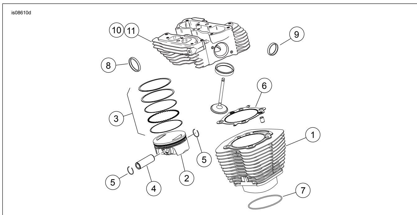
Slika 1. Servisni deli: Dirkalni komplet Screamin' Eagle Twin Cam 110 (1800 cc) Stage V
