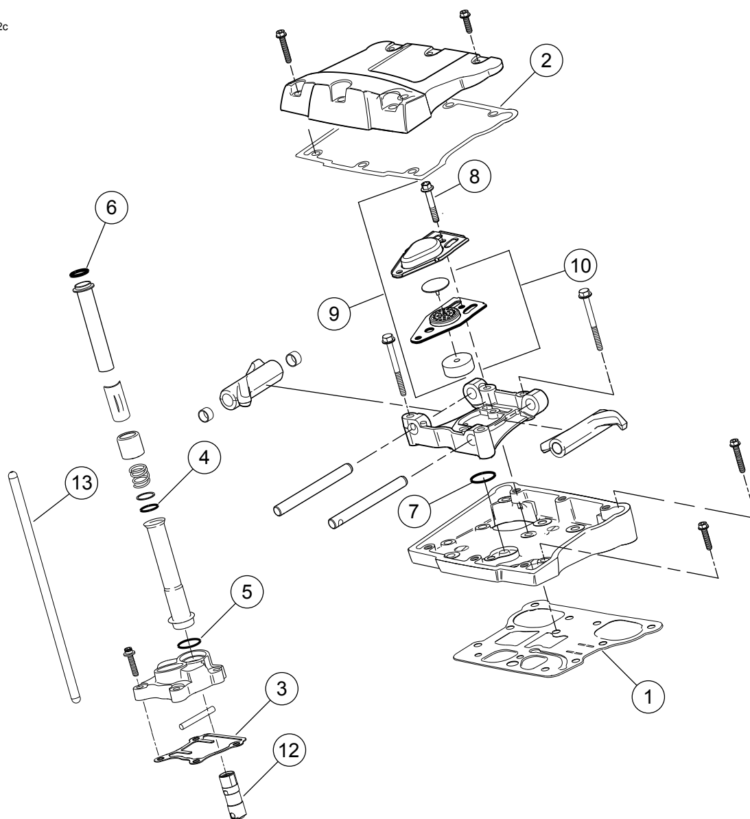
Slika 2. Servisni deli: Dirkalni komplet Screamin' Eagle Twin Cam 110 (1800 cc) Stage V
