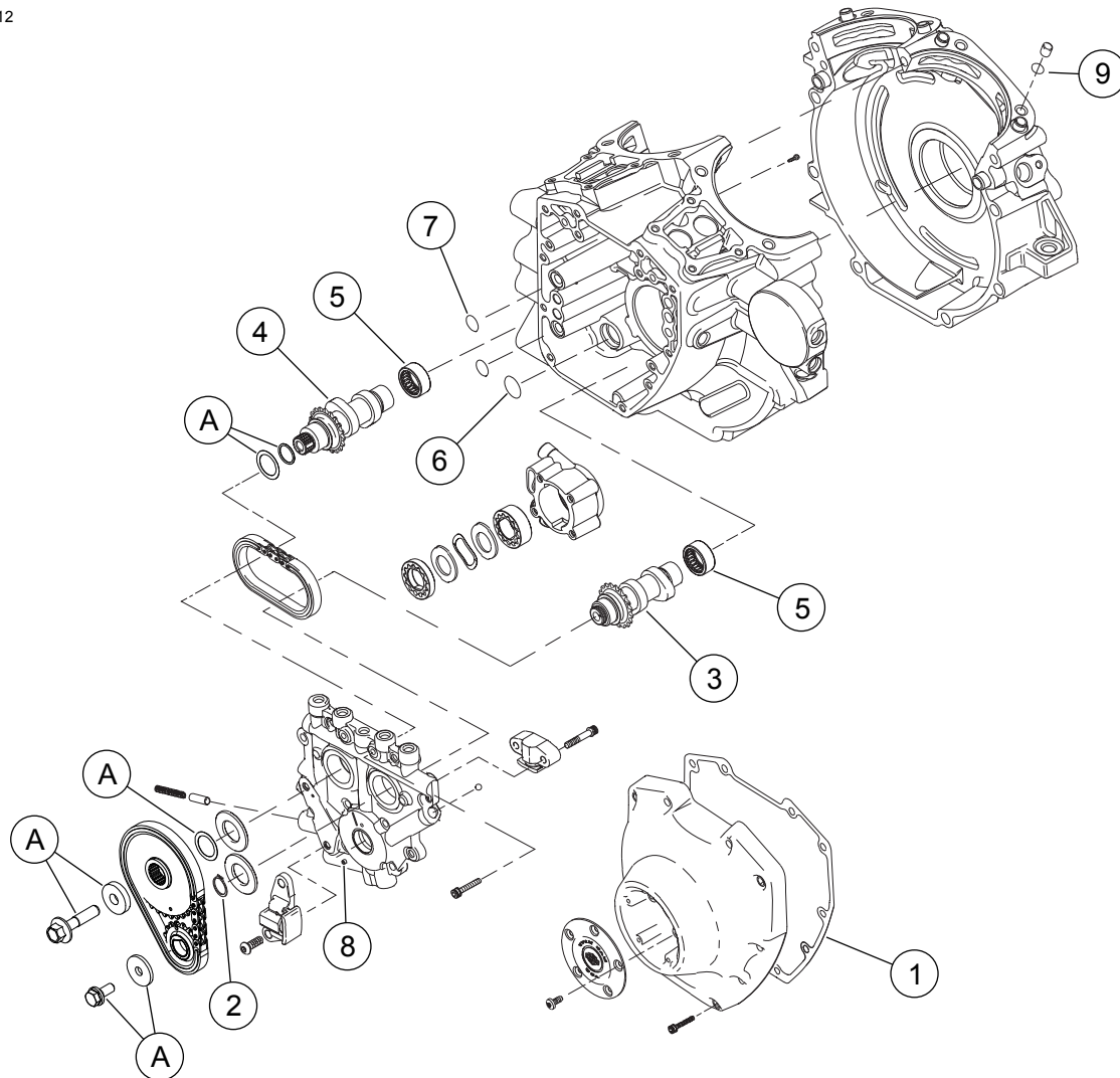
Pav 3. Dalys, reikalingos užduočiai atlikti "Screamin' Eagle Twin Cam 110" (1800 cc) V Etapo lenktynių komplektas
