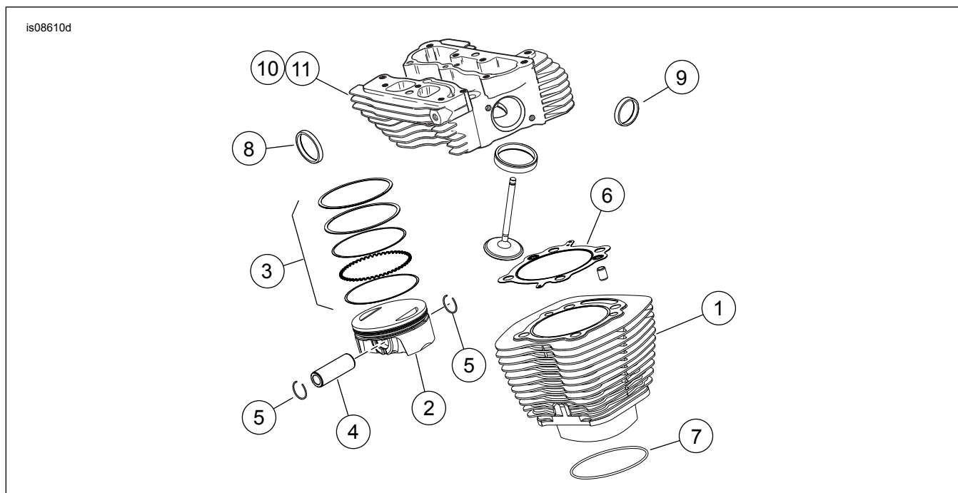
Pav 1. Dalys, reikalingos užduočiai atlikti "Screamin' Eagle Twin Cam 110" (1800 cc) V Etapo lenktynių komplektas
