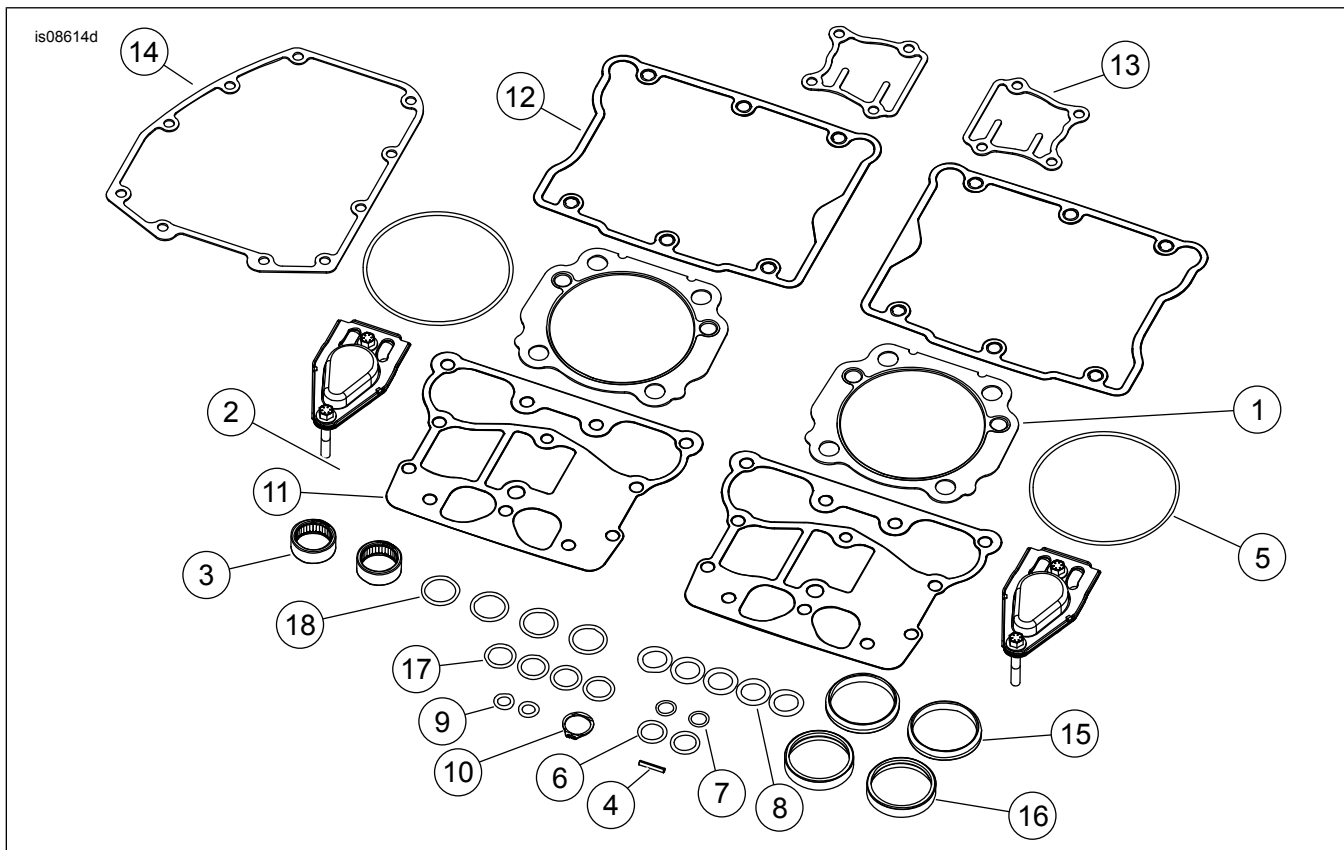
Pav 4. Dalys, reikalingos užduočiai atlikti "Screamin' Eagle Twin Cam 110" (1800 cc) V Etapo lenktynių komplektas
