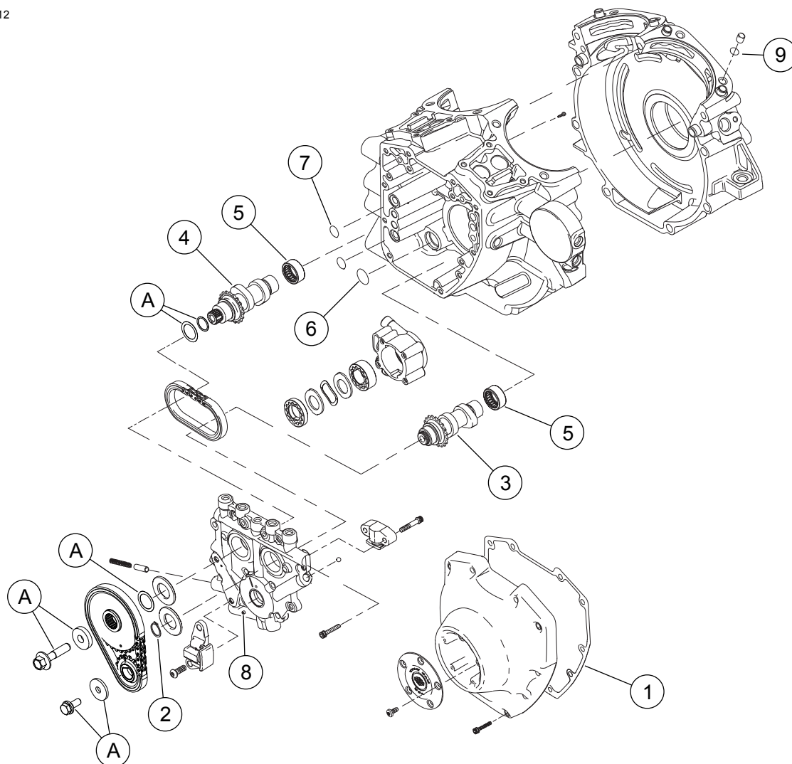
Slika 3. Servisni dijelovi: Screamin' Eagle Twin Cam 110 (1800 ccm) Stage V komplet za utrku
