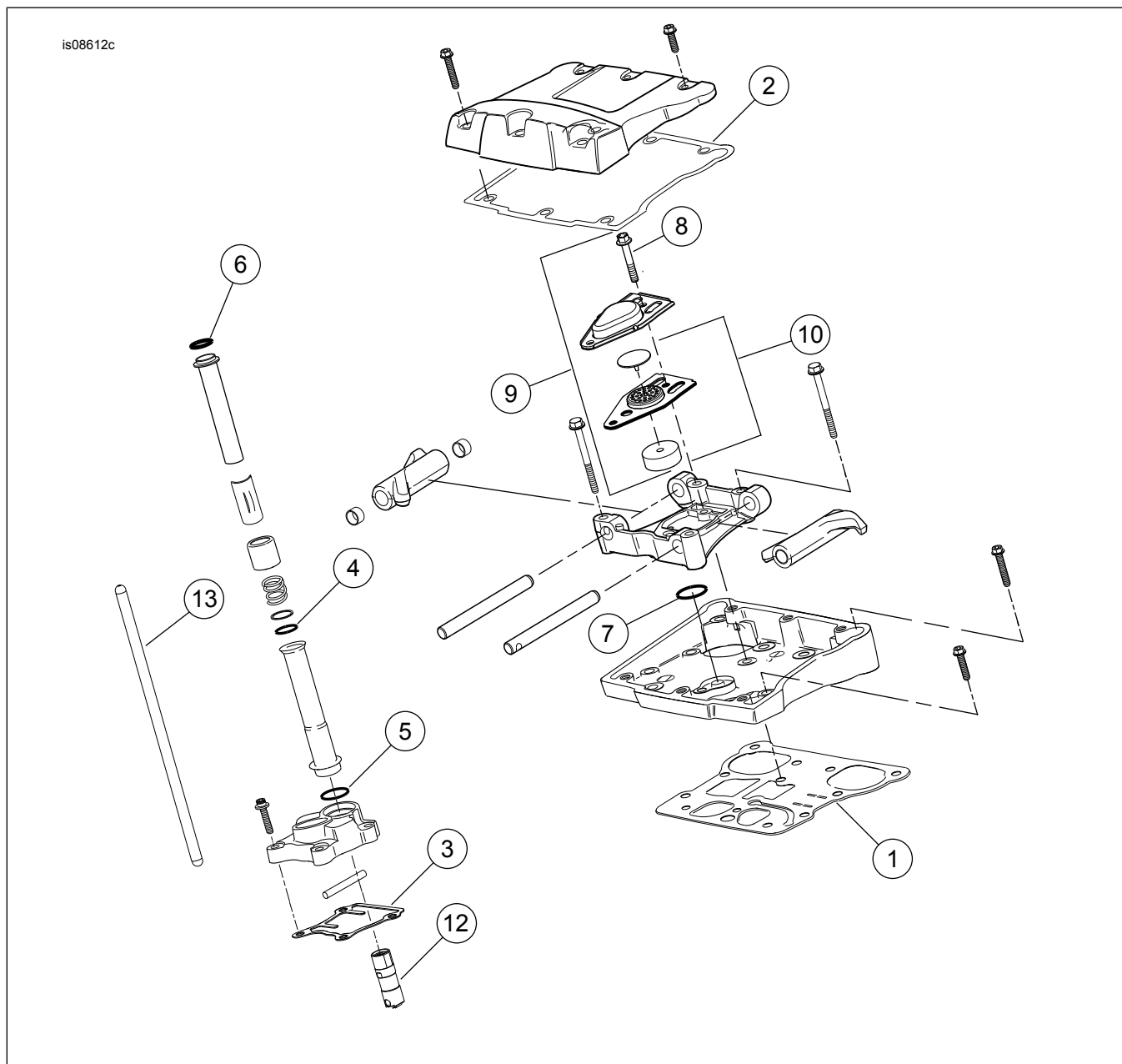
Slika 2. Servisni dijelovi: Screamin' Eagle Twin Cam 110 (1800 ccm) Stage V komplet za utrku
