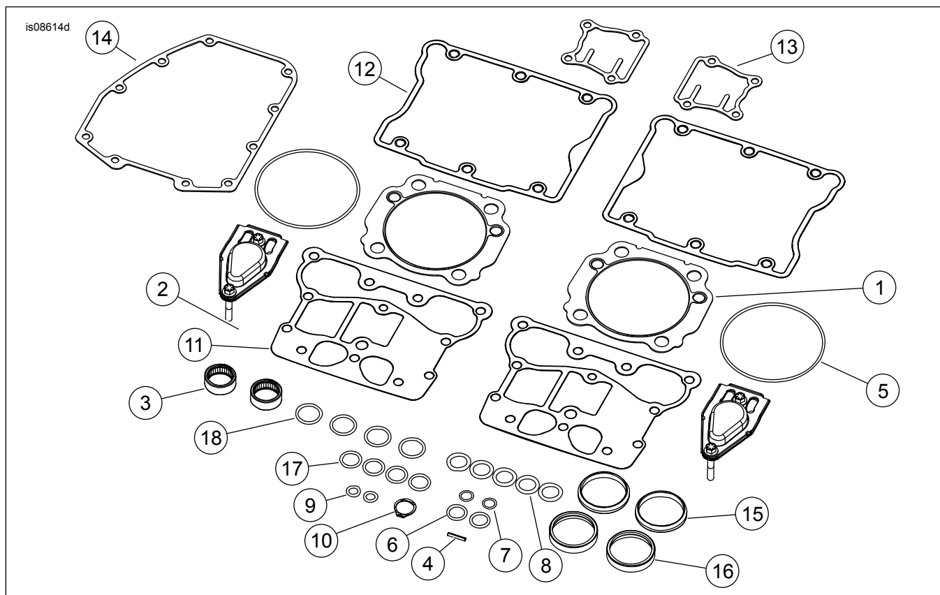
Slika 4. Servisni dijelovi: Screamin' Eagle Twin Cam 110 (1800 ccm) Stage V komplet za utrku
