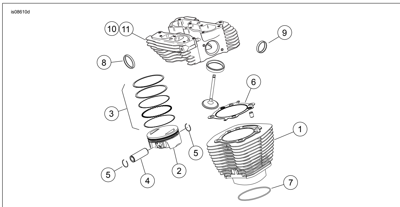
Slika 1. Servisni dijelovi: Screamin' Eagle Twin Cam 110 (1800 ccm) Stage V komplet za utrku
