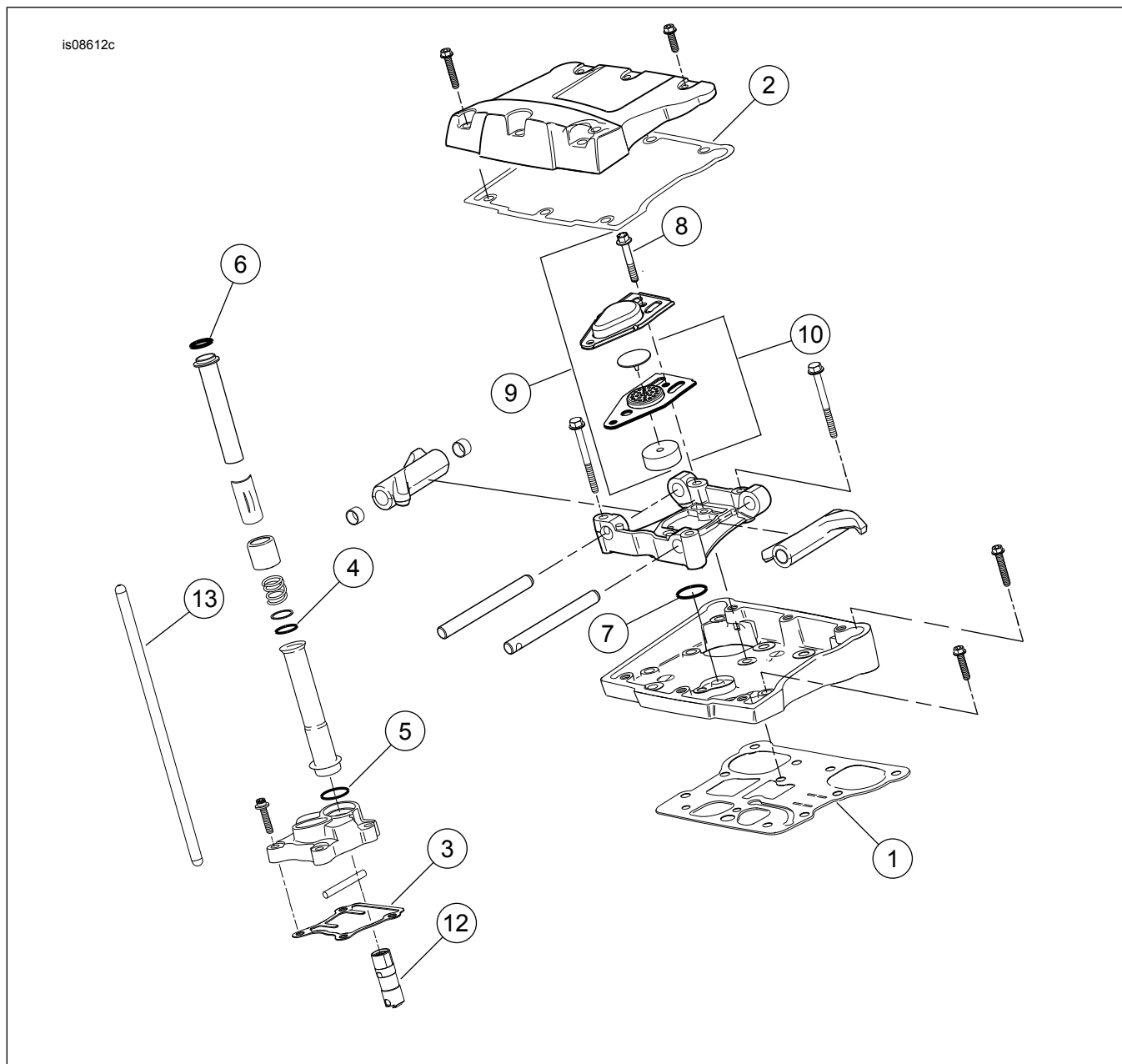
Afbeelding 2. Serviceonderdelen: Screamin' Eagle Twin Cam 110 (1800 cc) Stage V Race Kit
