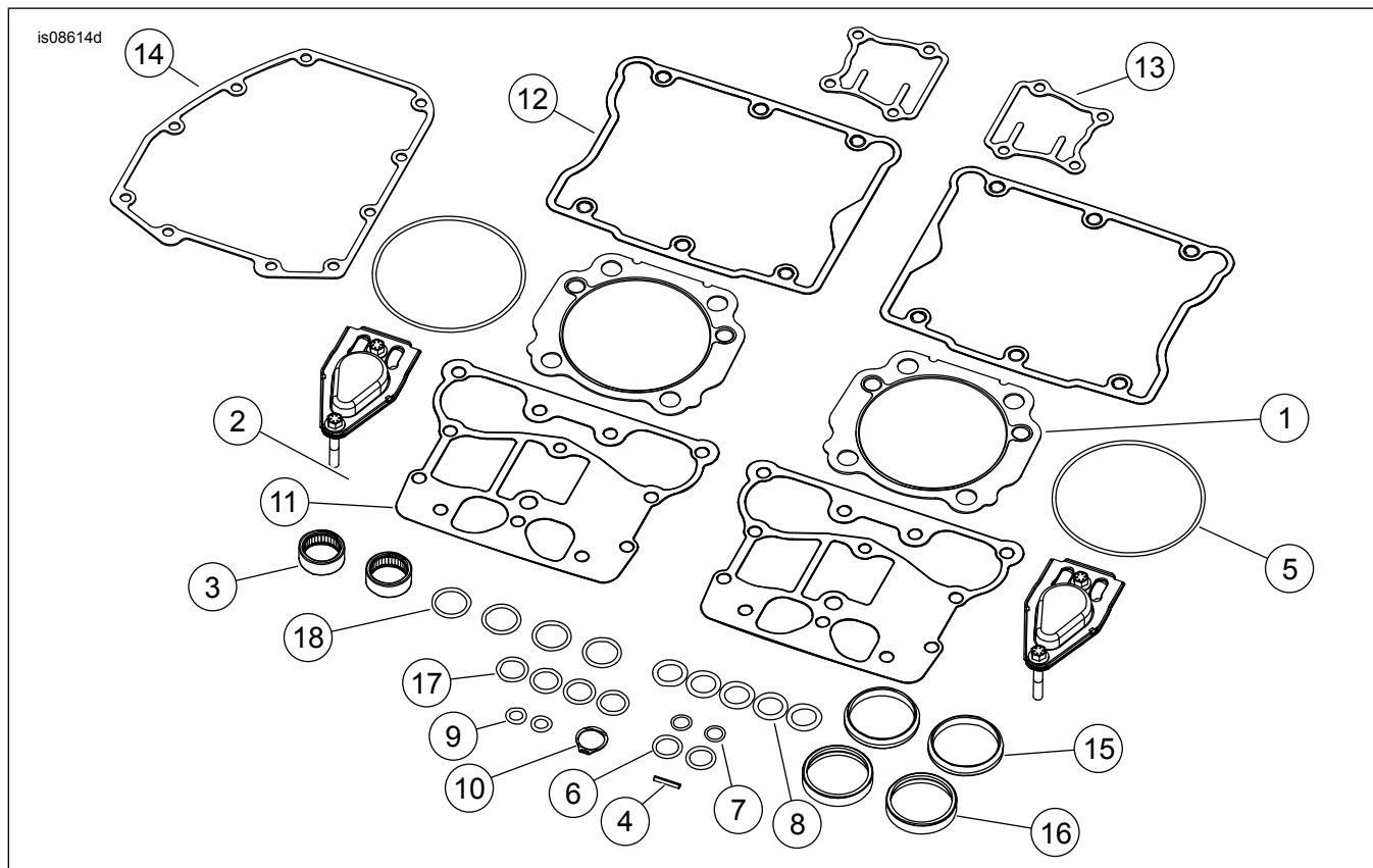
Afbeelding 4. Serviceonderdelen: Screamin' Eagle Twin Cam 110 (1800 cc) Stage V Race Kit
