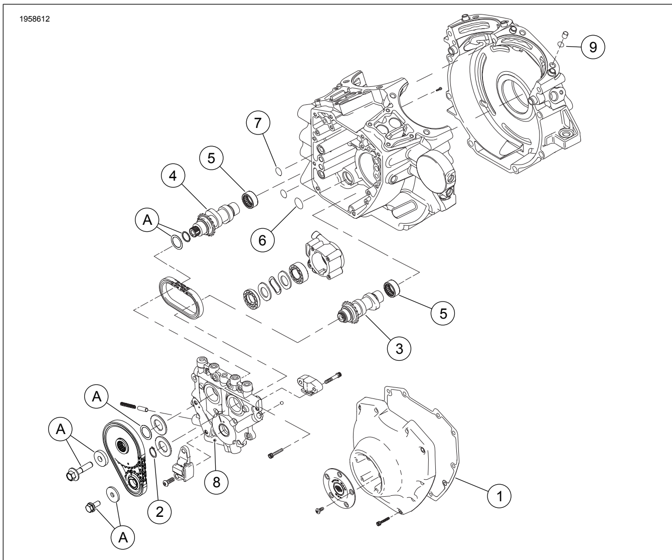
Afbeelding 3. Serviceonderdelen: Screamin' Eagle Twin Cam 110 (1800 cc) Stage V Race Kit
