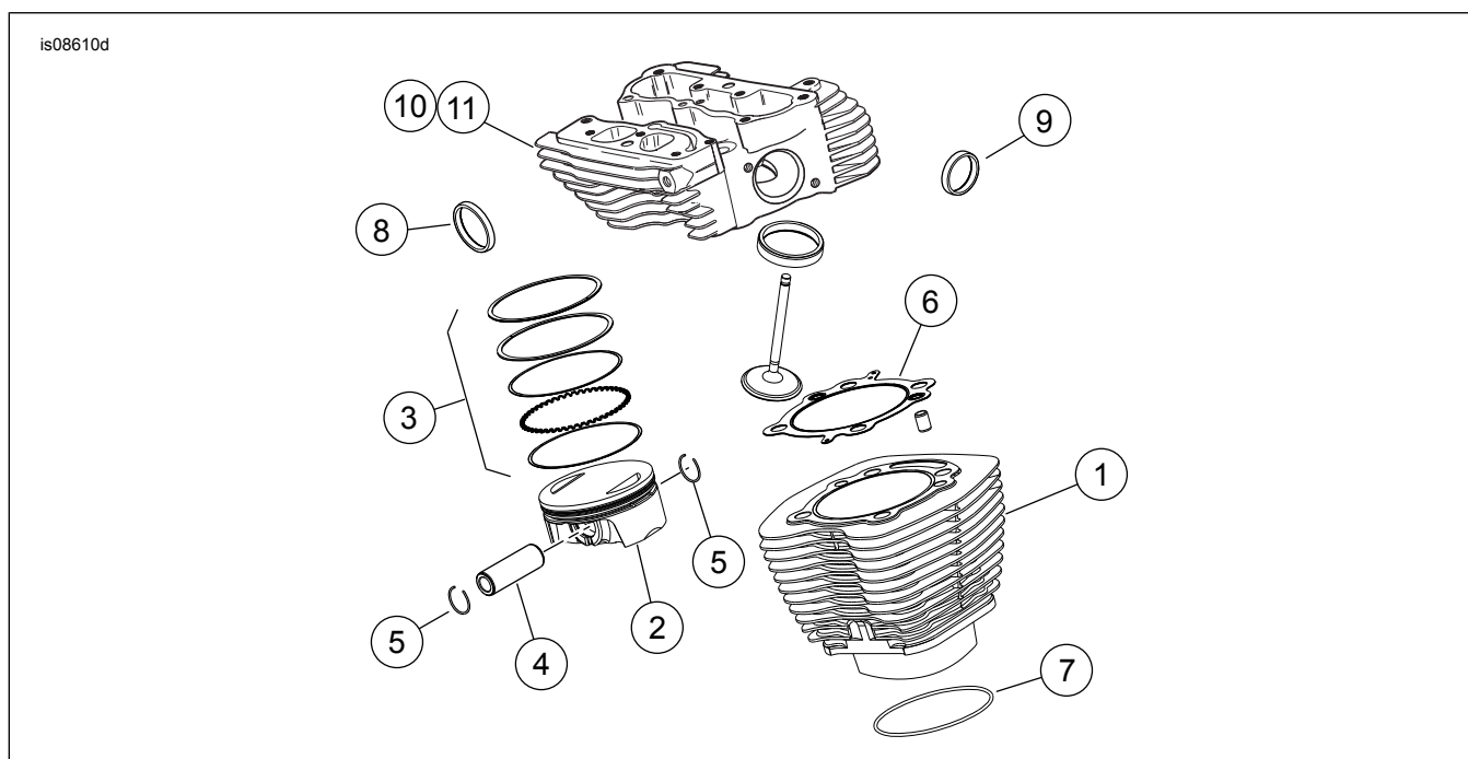
Afbeelding 1. Serviceonderdelen: Screamin' Eagle Twin Cam 110 (1800 cc) Stage V Race Kit
