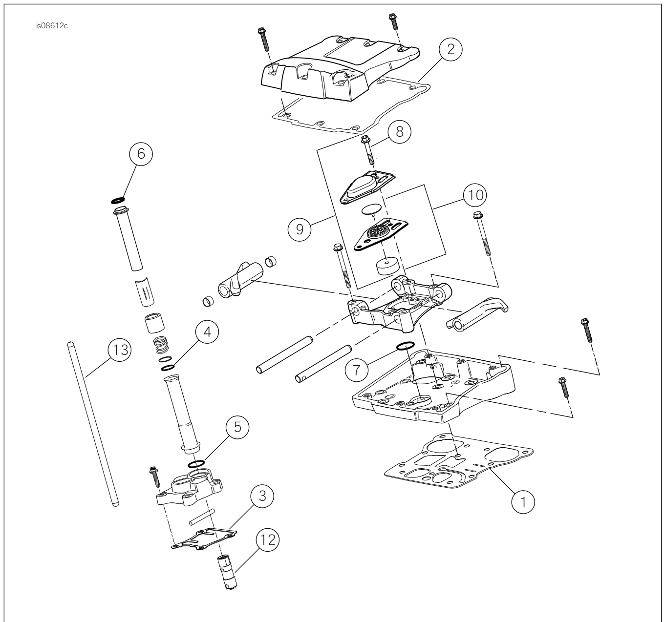
圖2。維修零件Screamin' EagleTwinCam110( 1800cc )StageV競賽級工具包
