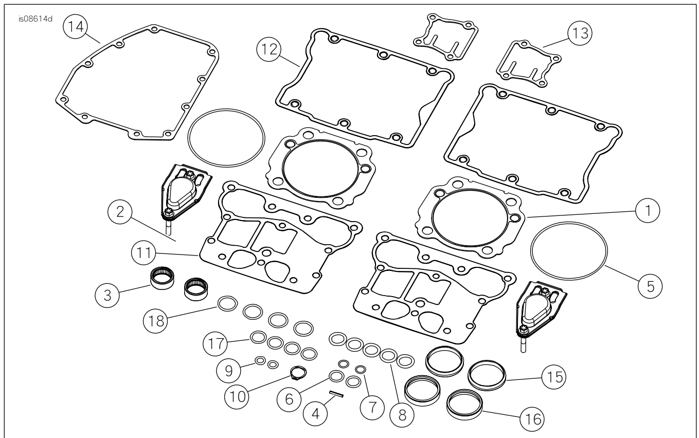
圖4。維修零件Screamin' EagleTwinCam110( 1800cc )StageV競賽級工具包
