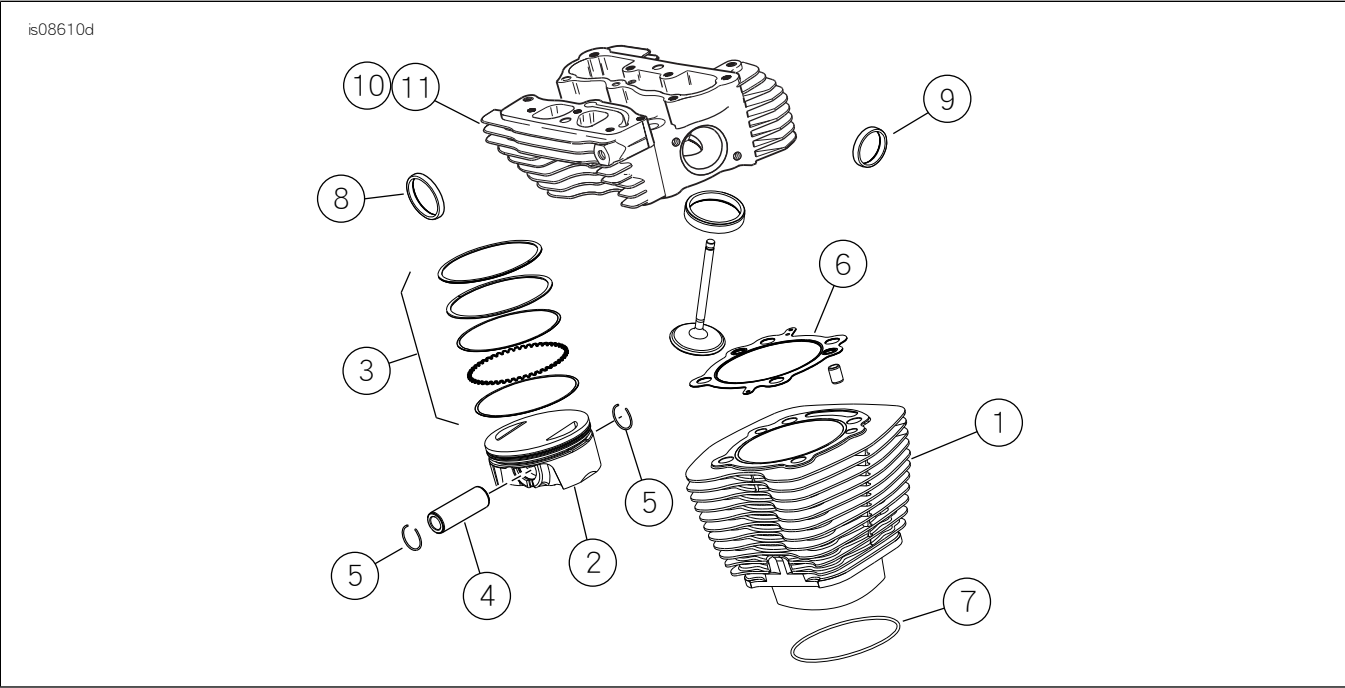
圖1。維修零件Screamin' EagleTwinCam110( 1800 cc )StageV競賽級工具包
