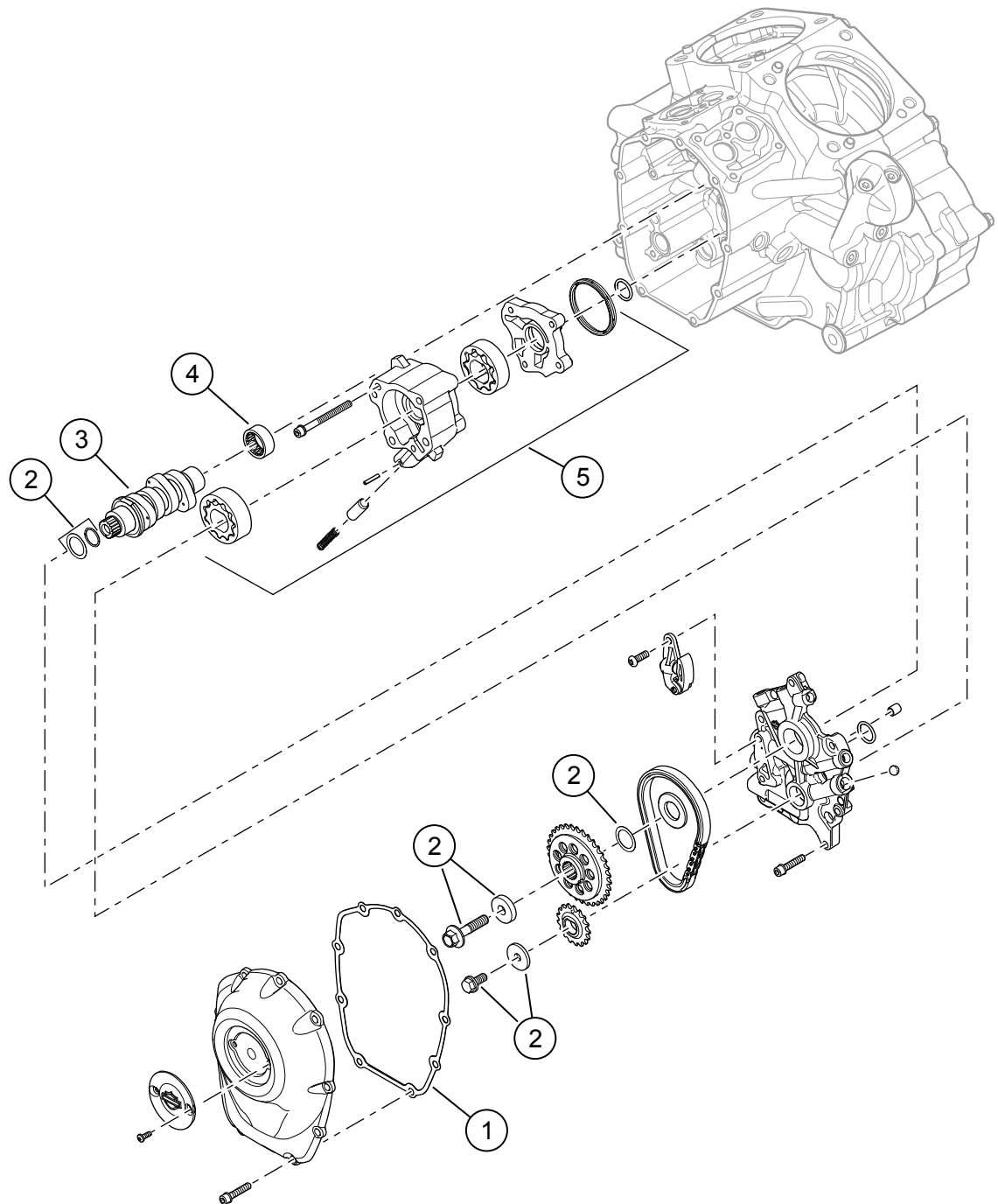
Ábra 2. Szervizelhető alkatrészek: Screamin' Eagle Milwaukee-eight Stage 2 készlet
