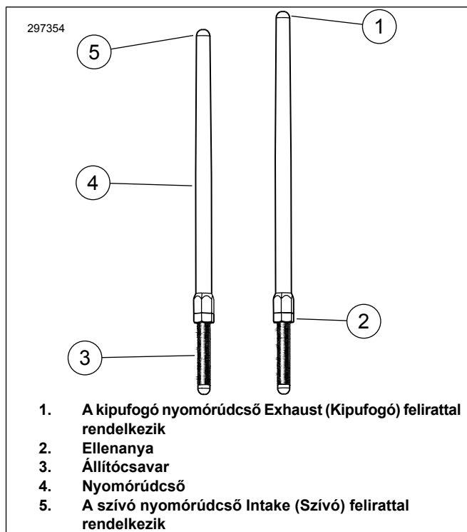
Ábra 3. Állítható nyomórúd
