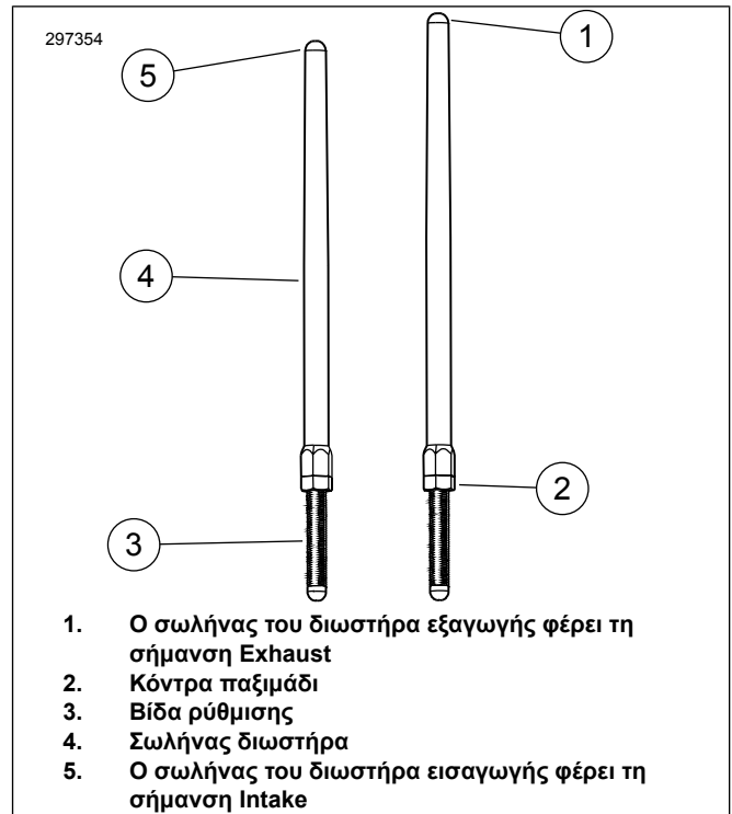
Εικόνα 3. Ρυθμιζόμενος διωστήρας
