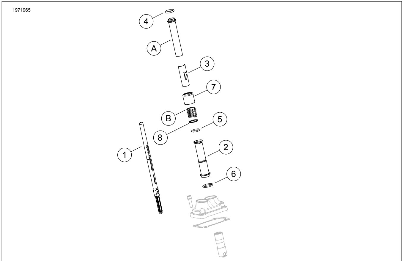
Εικόνα 1. Περιεχόμενα του κιτ: Κιτ Screamin' Eagle Milwaukee-Eight Βαθμίδας 2
