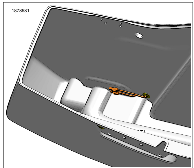
Фигура 4. Маршрутизиране на джъмперни окабелявания
