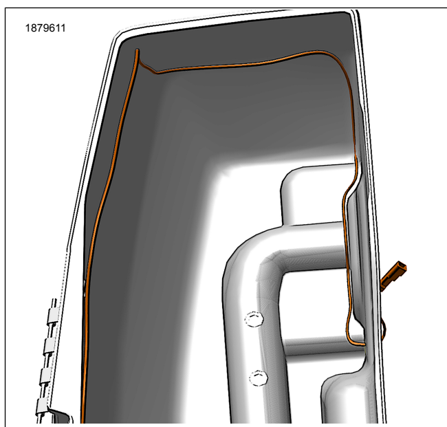
Фигура 7. Прокарване на окабеляване
