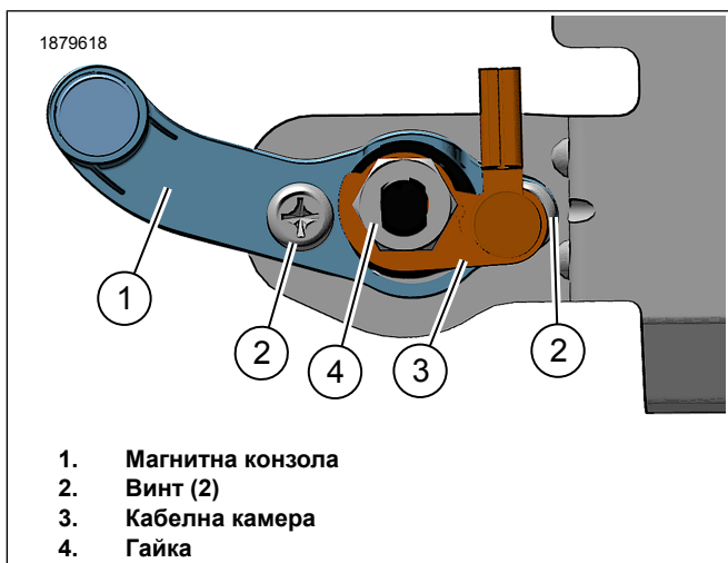
Фигура 5. Монтаж на магнитна конзола
