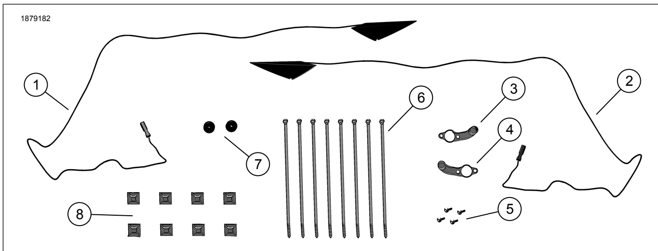
Фигура 1. Съдържание на комплекта: Вътрешно LED осветление за дисаги
