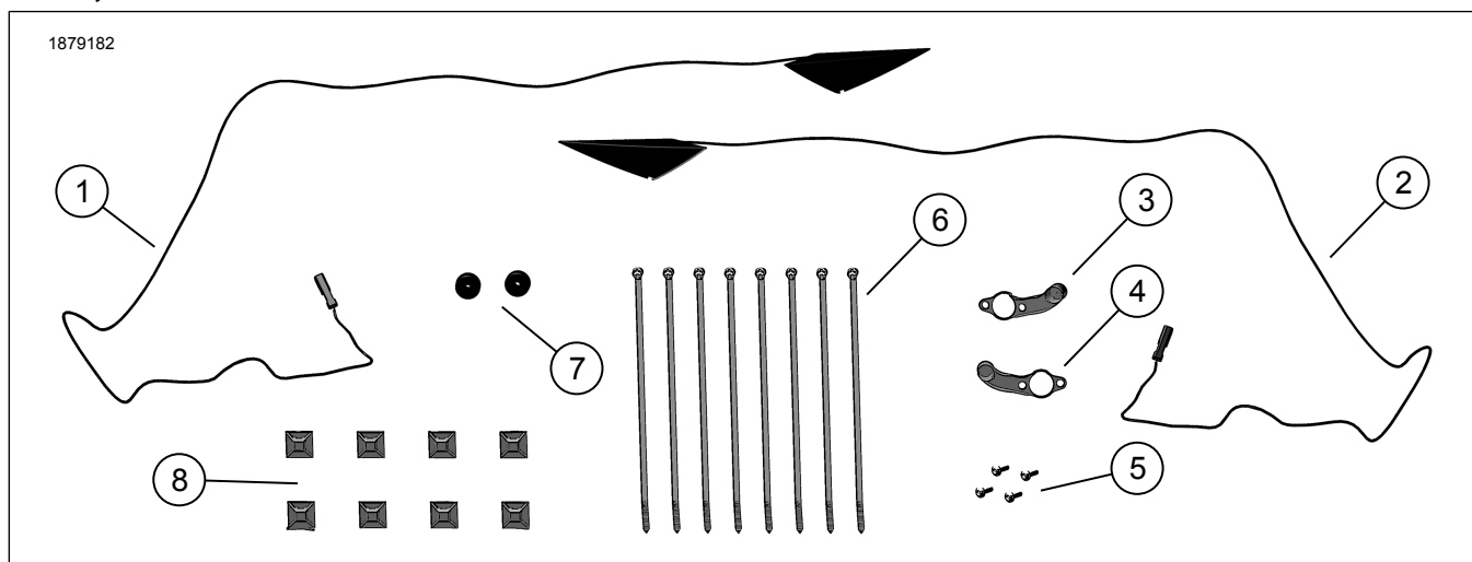
Figura 1. Conținut kit: Lumină interioară LED pentru desagă
