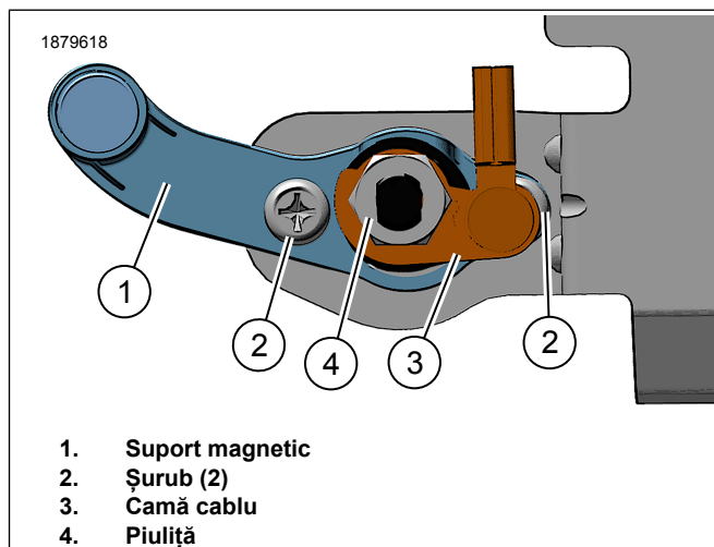
Figura 5. Ansamblu suport magnetic
