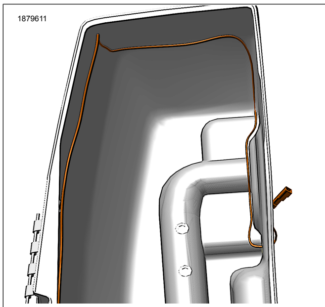
Attēls 7 Savienotājkabeļa maršrutēšana
