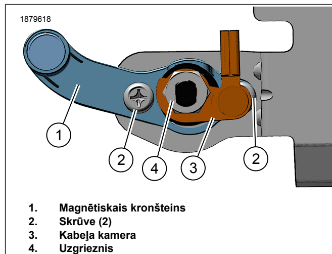
Attēls 5 Magnētiskā kronšteina mezgls
