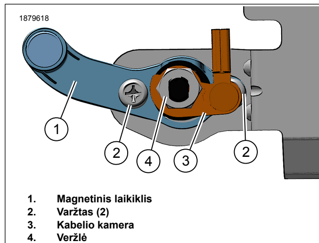
Pav 5. Magnetinio laikiklio surinkimas
