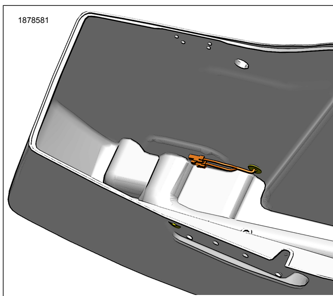
Obrázok 4. Vedenie zväzku prepojky
