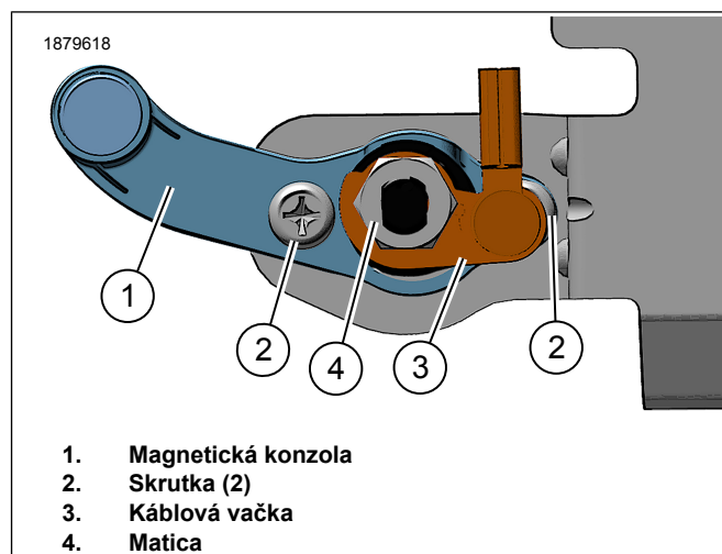
Obrázok 5. Zostava magnetickej konzoly
