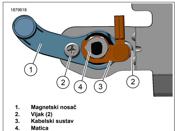
Slika 5. Sklop magnetskog nosača
