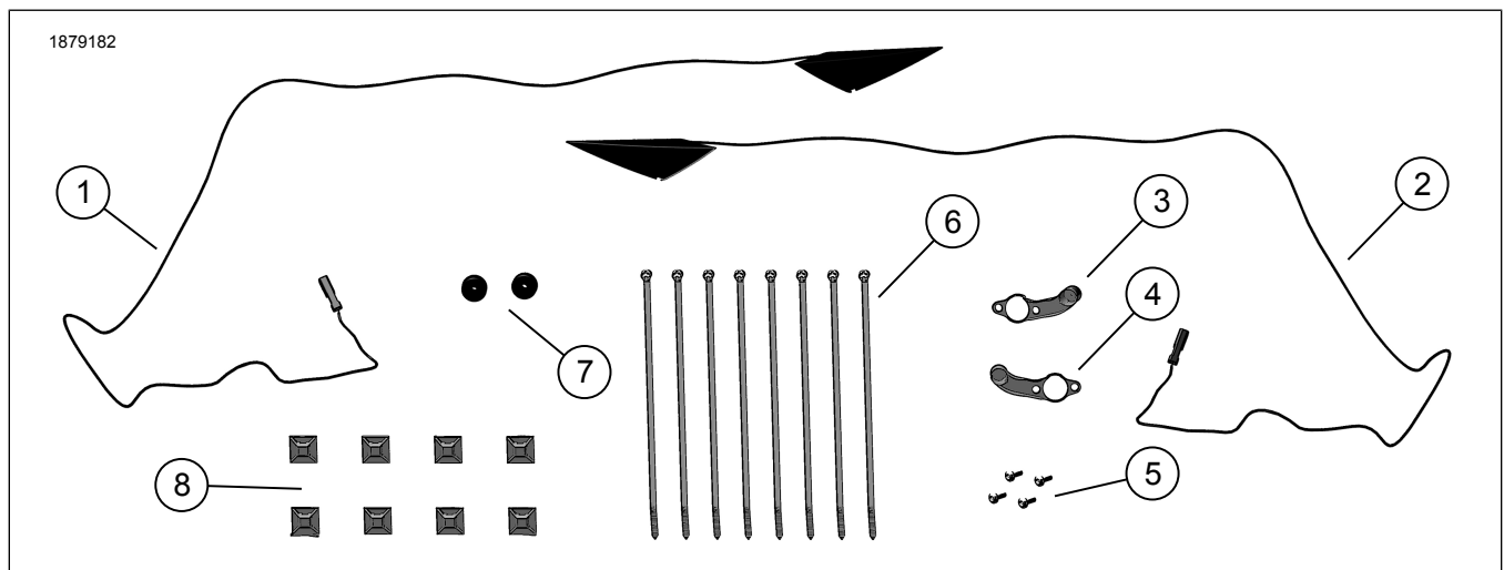
Slika 1. Sadržaj kompleta: Unutarnje LED svjetlo torbe za sjedalo
