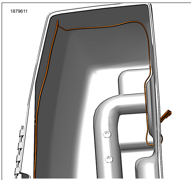
Figur 7. Trekking av ledningsselle
