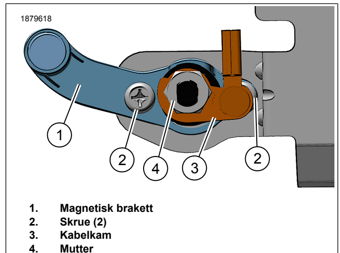
Figur 5. Magnetisk brakettenhet
