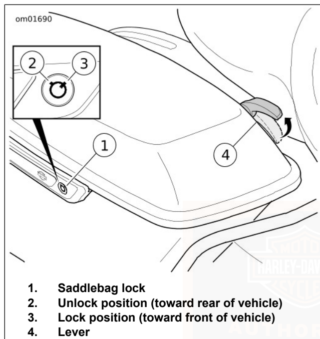
Figure 56. Saddlebag
