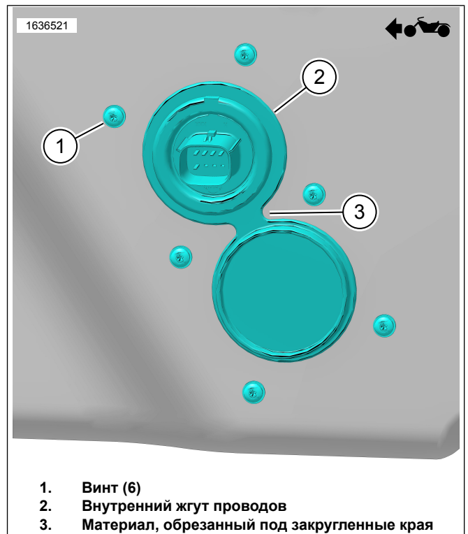
Рисунок 7. Панель внутреннего жгута проводов
