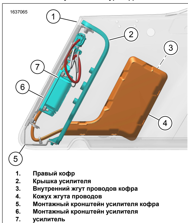
Рисунок 13. Жгут проводов кофра с усилителем
