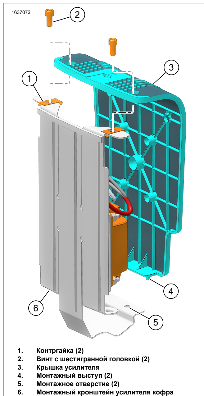
Рисунок 14. Крышка усилителя
