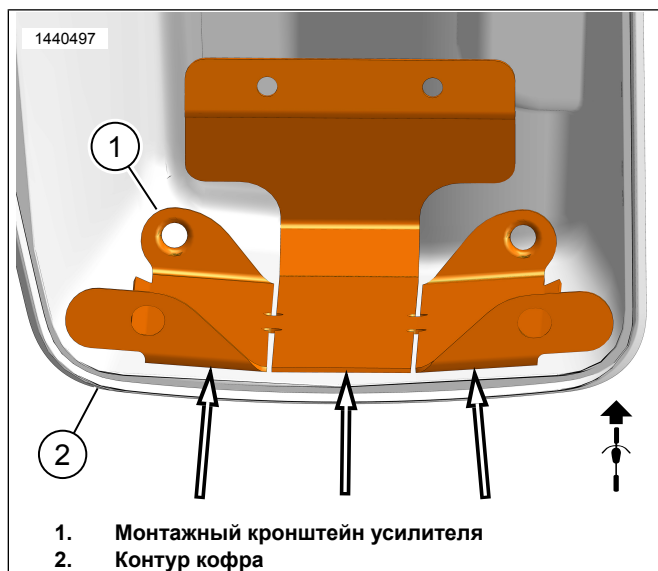
Рисунок 12. Контур кофра
