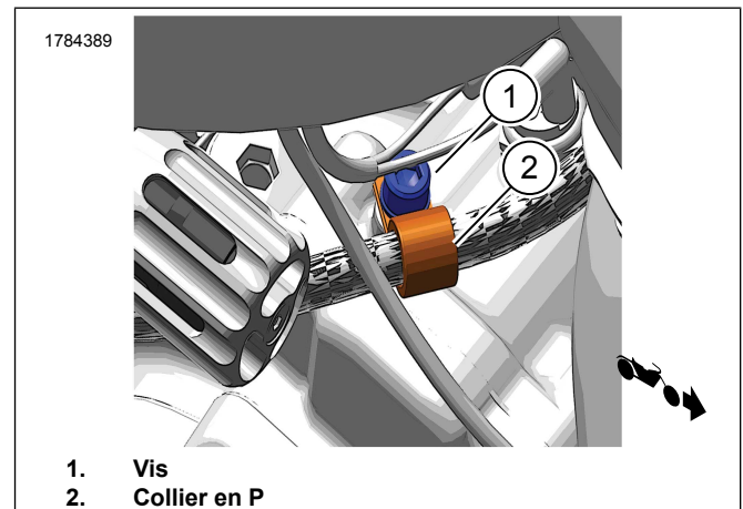
Figure 2. Installer le collier en P et la vis
