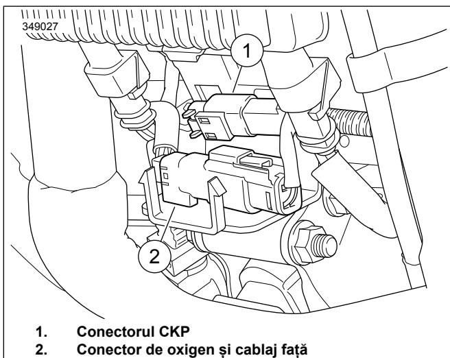
1. Conectorul CKP 2. Conector de oxigen și cablaj față Figura 39. Locația senzorului de oxigen față
