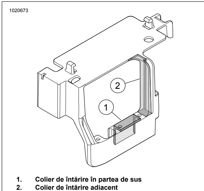
Figura 28. Zonele evidențiate pentru a fi tăiate
