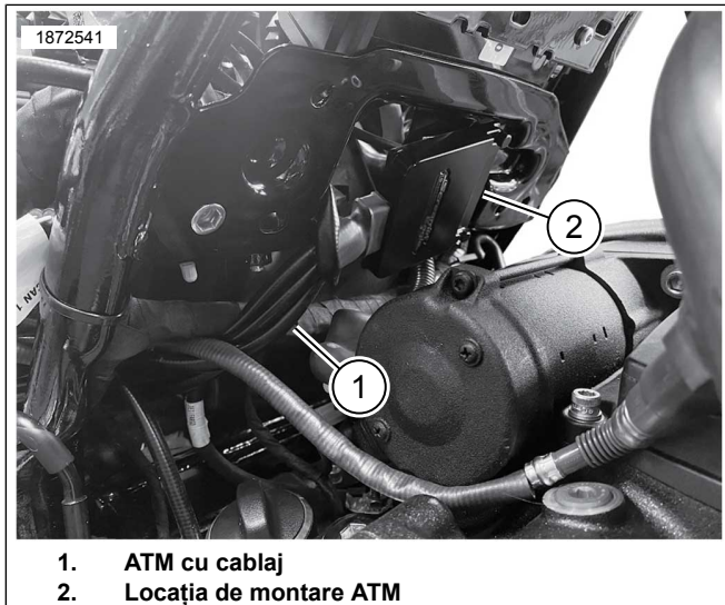
Figura 5. Locația de montare ATM
