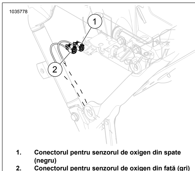
Figura 1. Locația senzorului de oxigen din spate și din față
