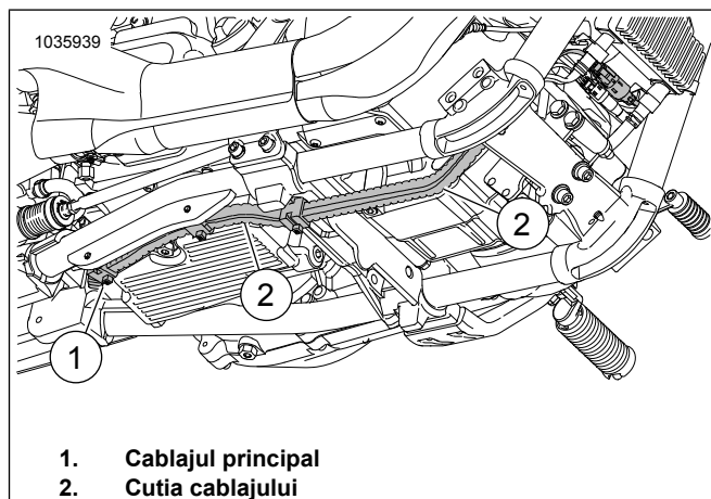
Figura 44. Cutia cablajului
