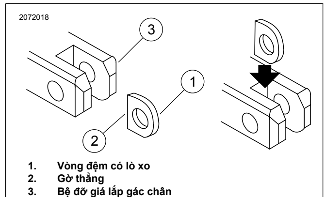
Hình 3. Lắp vòng đệm có lò xo của góc chân
