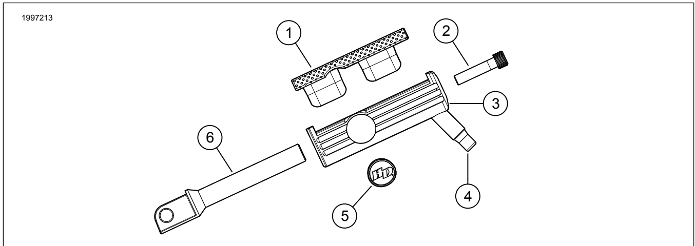
Hình 1. Các chi tiết trong bộ sản phẩm: Phụ tùng không chính hãng
