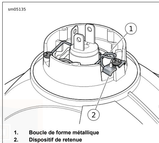
Figure 61. Ensemble d'ampoule du phare
