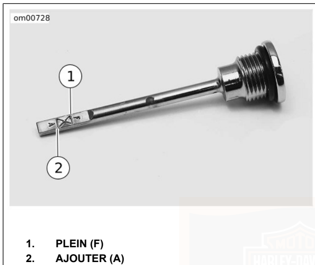
Figure 51. Niveau du lubrifiant du bouchon de remplissage/jauge de la transmission
