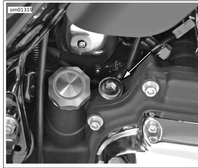
Figure 50. Emplacement du bouchon de remplissage/jauge de la transmission
