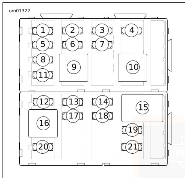
Figure 75. Fusibles : Modèles Tri Glide
