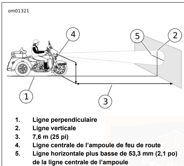
Figure 62. Vérifier l'alignement du phare
