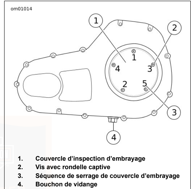
Figure 52. Couvercle du carter de chaîne primaire
