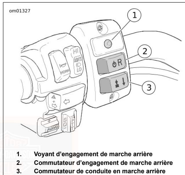
Figure 23. Commandes de marche arrière
