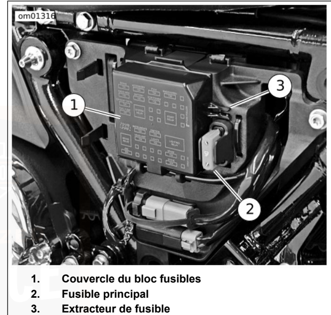
Figure 74. Bloc fusibles : Modèles Tri Glide
