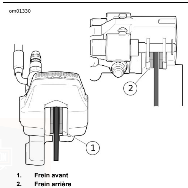
Figure 54. Matériau de friction des freins : Modèles Tri Glide
