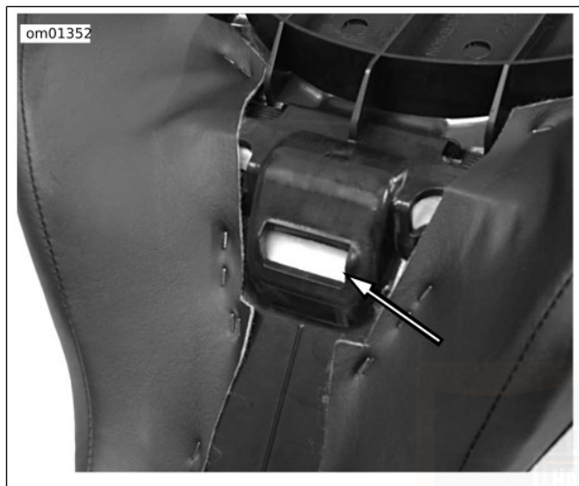
Figure 78. Fente de la selle : Modèles Tri Glide BOUCLES DE POINTS D'ATTACHE DE L'ESSIEU ARRIÈRE
