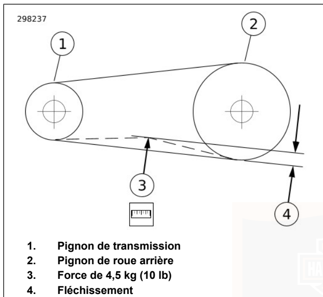
Figure 53. Vérifier le fléchissement de la courroie
