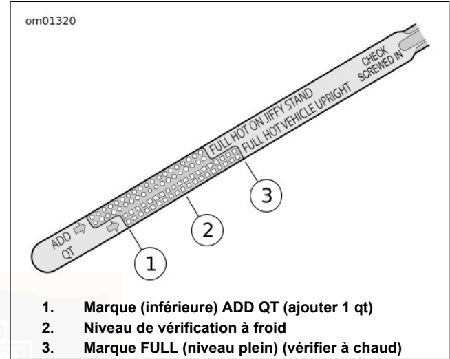
Figure 46. Jauge de l'huile moteur
