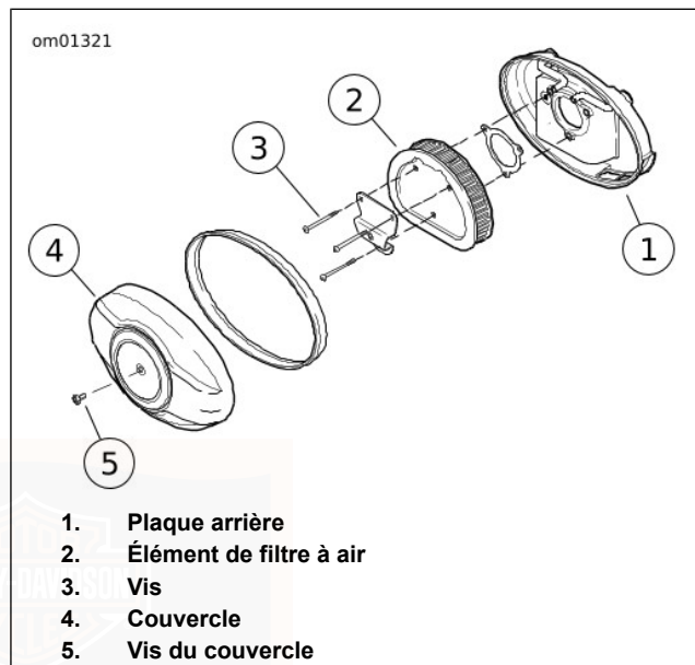
Figure 60. Filtre à air : Modèles Twin Cam
