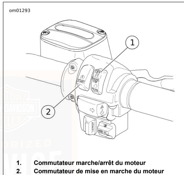
Figure 42. Commandes sur la droite du guidon
