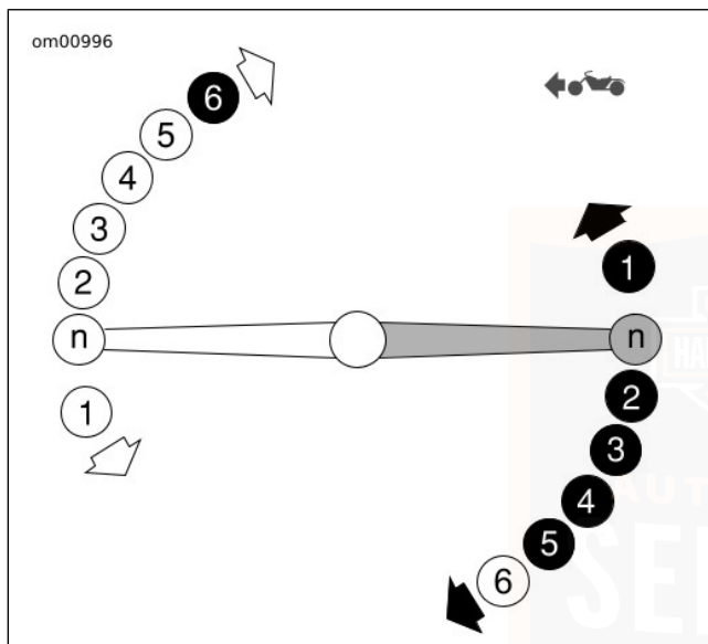
Figure 11. Pédale de sélection de vitesse talon/pointe
