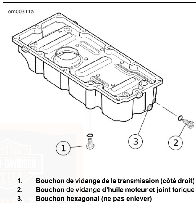
Figure 47. Carter d'huile
