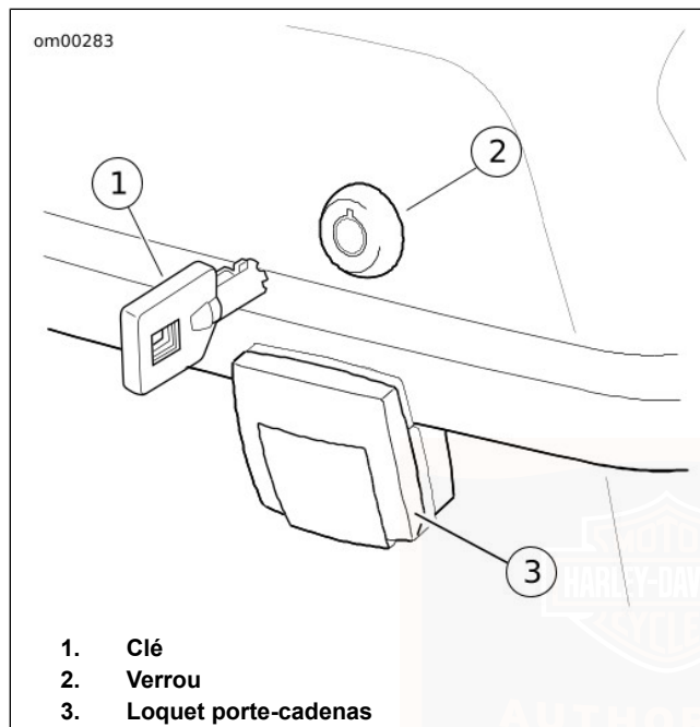
Figure 14. Verrou et loquet porte-cadenas du coffre Tour-Pak
