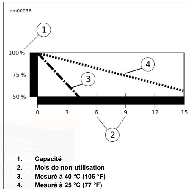
Figure 70. Effet de la température sur la vitesse de décharge spontanée d'une batterie
