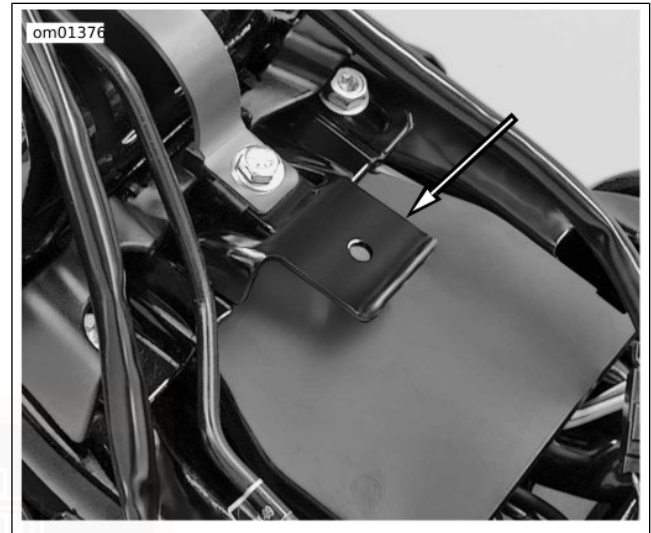
Figure 77. Languette de selle
