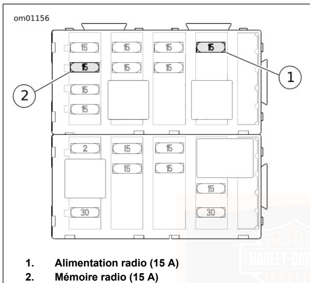
Figure 35. Fusibles de radio
