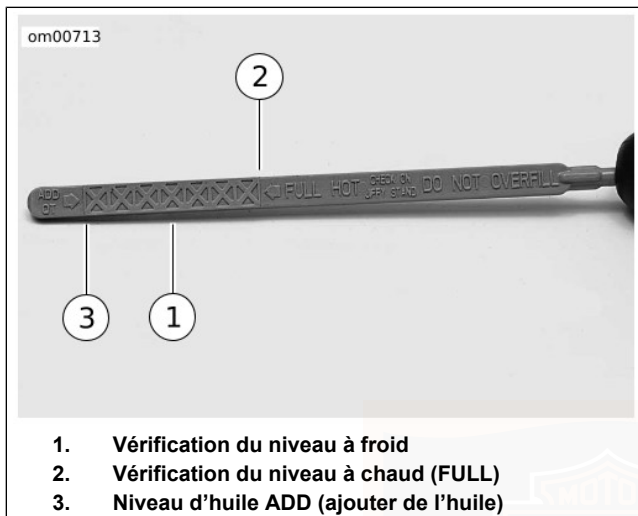
Figure 22. Niveau d'huile moteur : modèles Dyna CHANGEMENT D'HUILE ET DE FILTRE À HUILE : MODÈLES DYNA
