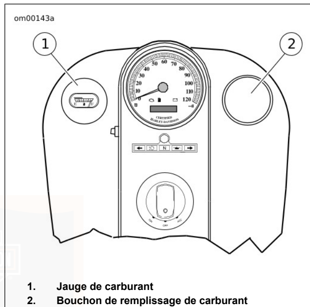
Figure 10. Jauge de carburant et bouchon de remplissage de carburant : modèles FXDL, FXDWG, FXDC et FXDB
