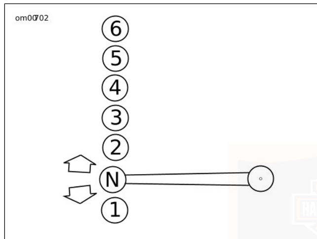
Figure 9. Grille de sélection de rapports
