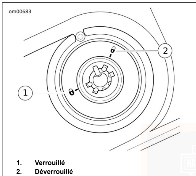
Figure 4. Verrou de fourche : FXDWG, FXDC
