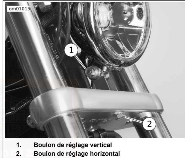
Figure 39. Réglage du phare
