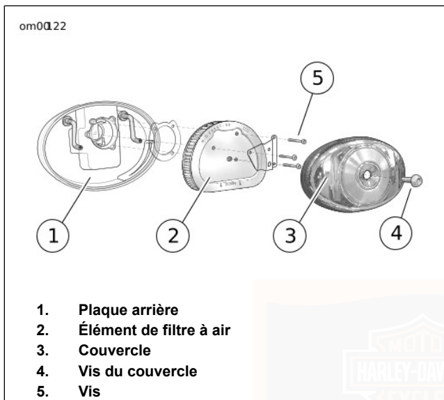
Figure 35. Épurateur d'air : modèles Twin Cam PHARE
