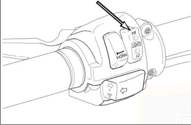
Figure 38. Commutateur du phare, réglage de feu de route
