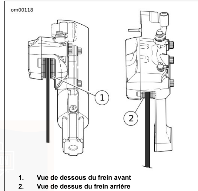
Figure 32. Mesure des plaquettes de frein externes PNEUS
