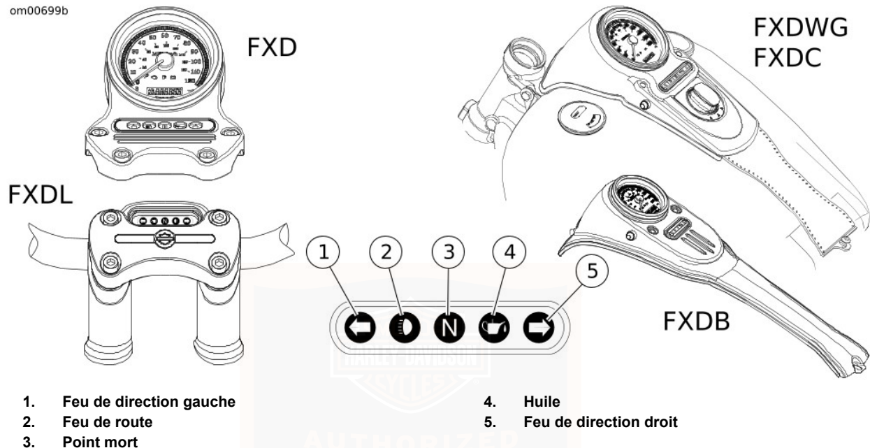
Figure 6. Indicateurs lumineux
