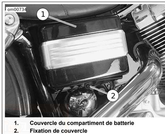
Figure 44. Compartiment de batterie : modèles Dyna DÉMARRAGE PAR CÂBLES
