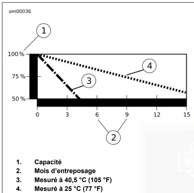
Figure 43. Effet de la température sur la vitesse de décharge spontanée d'une batterie
