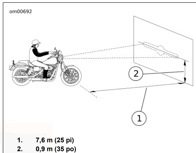
Figure 37. Vérification de l'alignement du phare : modèles Dyna
