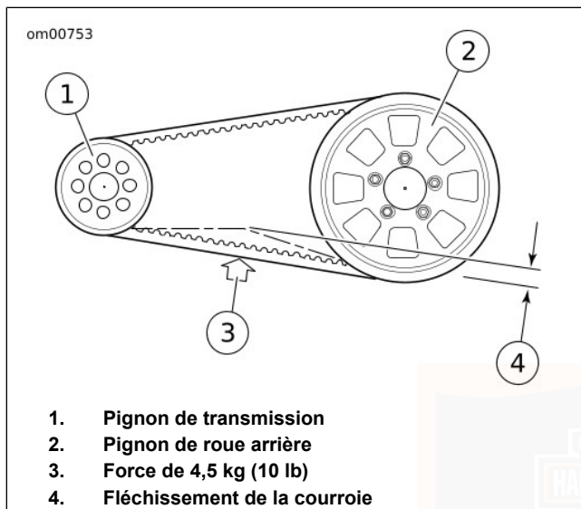
Figure 31. Fléchissement de la courroie : Modèles Dyna
