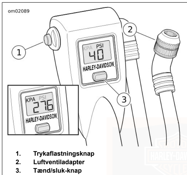
Figur 27. Digital Touring affjedringsluftpumpe
