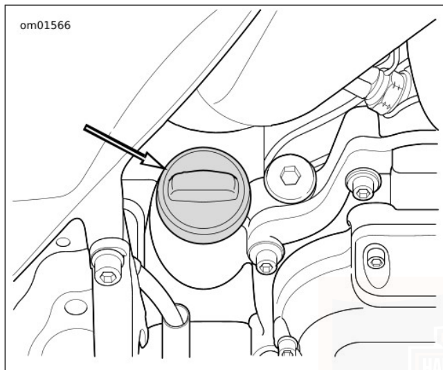
Figur 46. Motorens oliepåfyldningsprop
