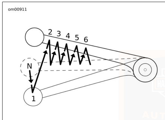
Figur 43. Gearskiftesekvens: Skift til højere gear
