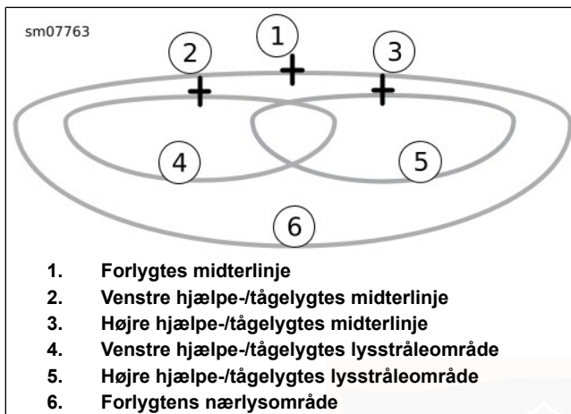
Figur 84. Forlygtemønster: LED-type med hjælpe-/tågelygter
