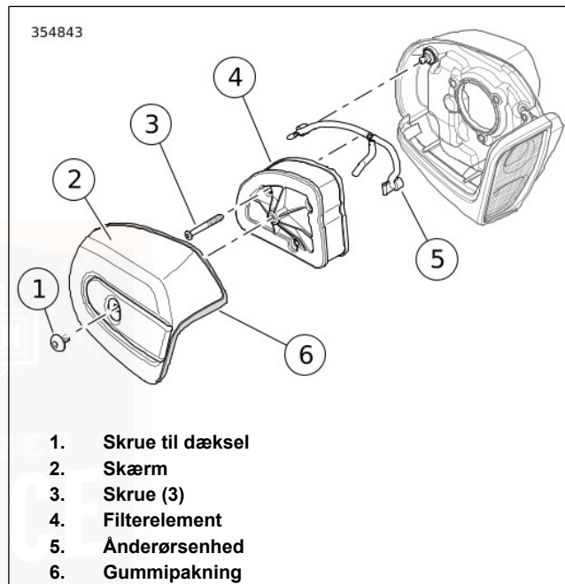
Figur 73. Luftrenser
