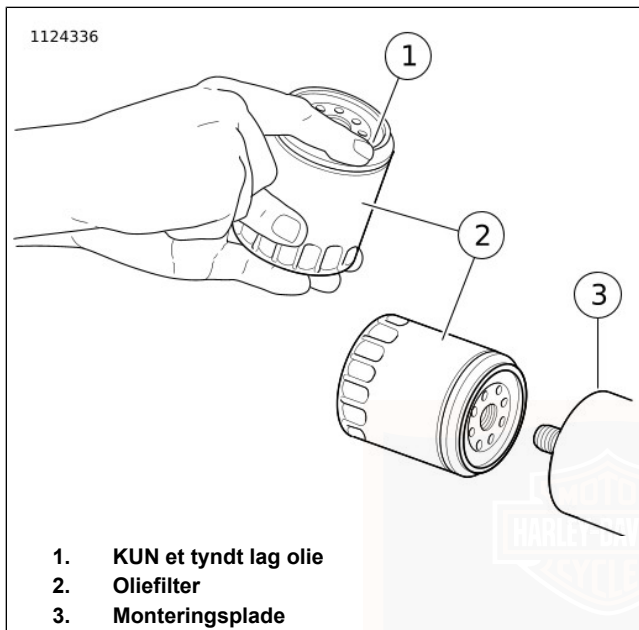
Figur 49. Påføring af en tynd oliefilm SMØRING VED LAV TEMPERATUR
