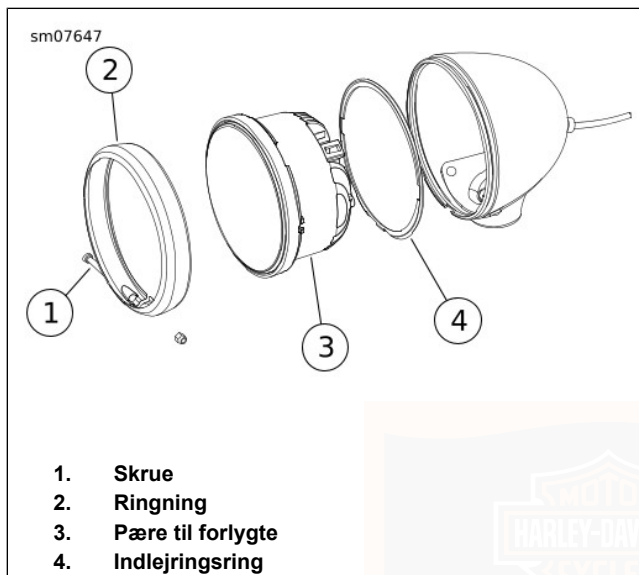
Figur 81. Forlygtemodul
