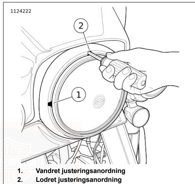
Figur 79. Forlygtens justeringsanordninger: Alle undtagen rammemonteret strømlinebeklædning (typisk)
