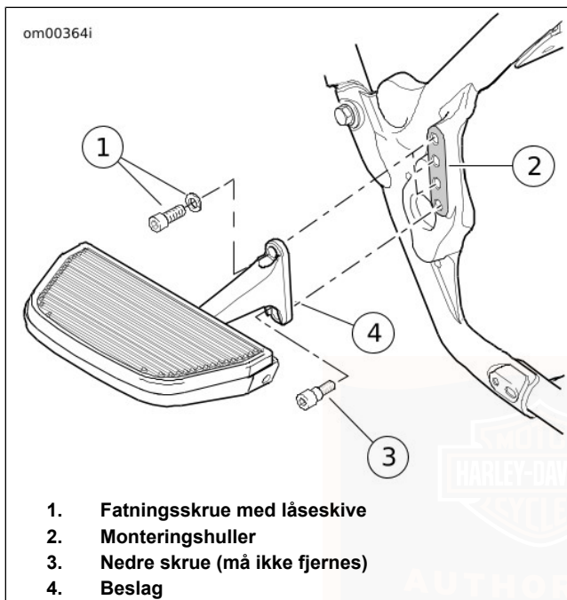
Figur 23. Passagerens fodstøtte
