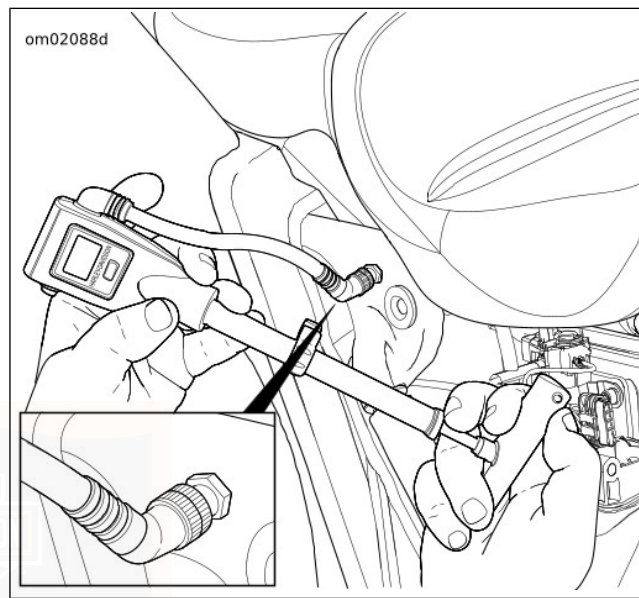
Figur 28. Justering af støddæmpers lufttryk
