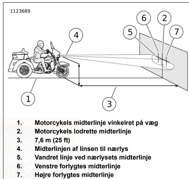
Figur 82. Forlygtejustering: To lysdioder
