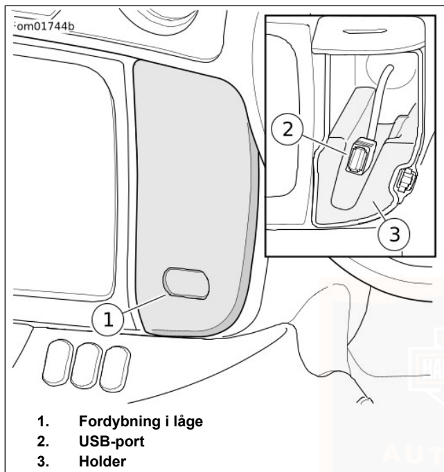
Figur 17. Medierum
