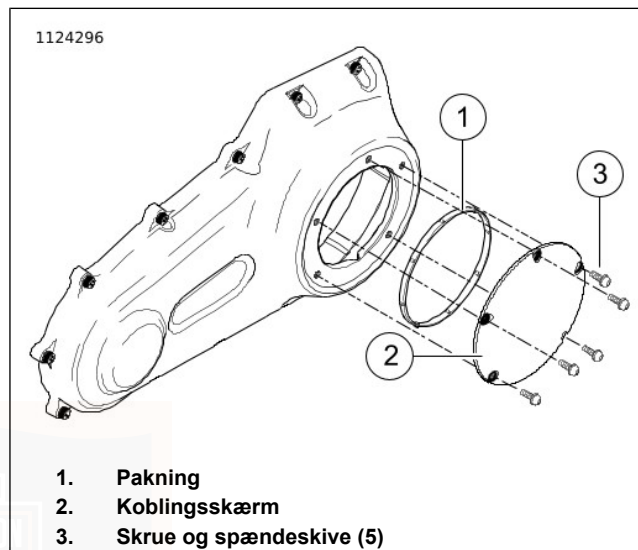
Figur 55. Koblingskærm (typisk)
