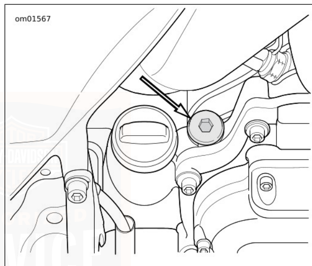
Figur 50. Placering af påfyldningsdæksel/oliepind til transmissionen
