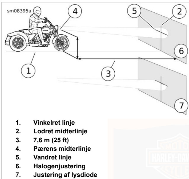
Figur 76. Forlygtejustering: FLRT, enkelt forlygte
