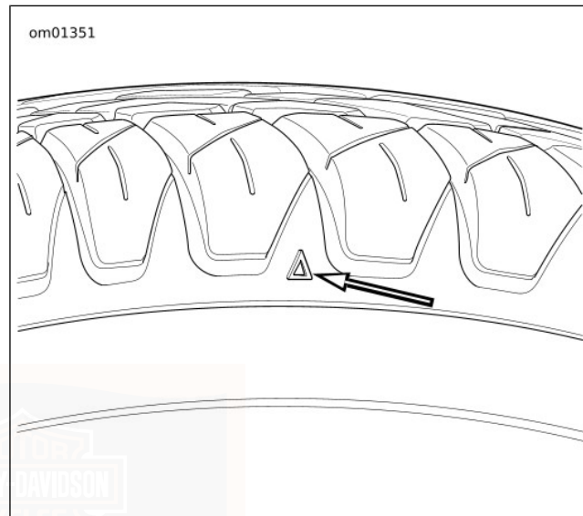
Figur 71. Slidbaneindikator på bageste dæk
