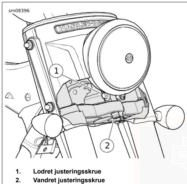
Figur 77. Justering af forlygte: FLRT
