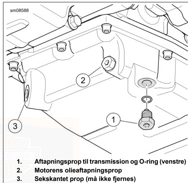
Figur 52. Udtømning af transmissionsvæske
