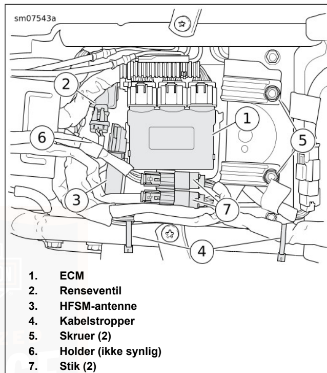
Figur 90. Øverste bakke
