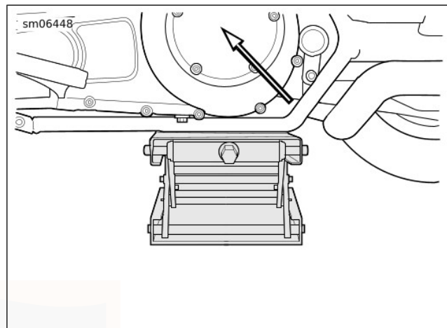
Figur 75. Placering af donkraft til løft af bagende
