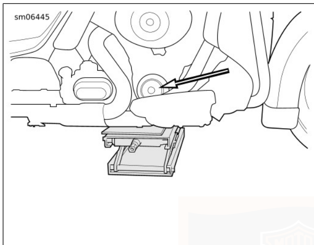
Figur 74. Placering af donkraft til løft af forende
