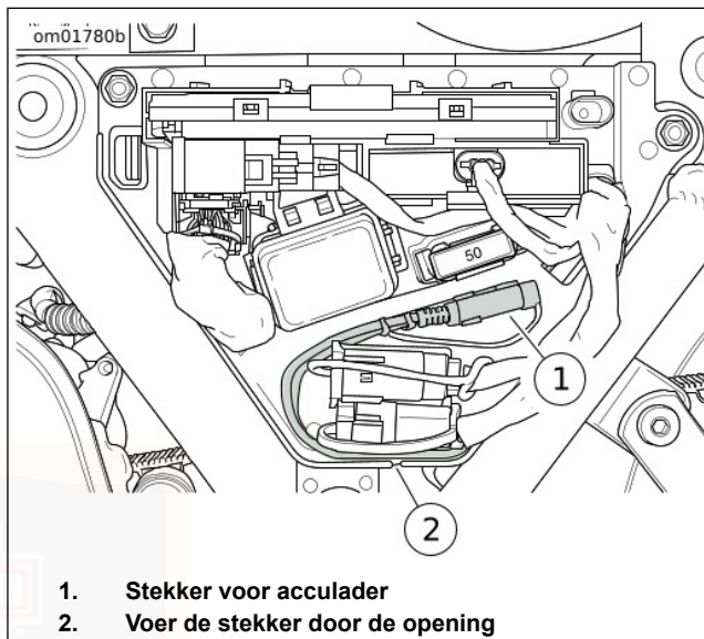
Afbeelding 76. Stekker acculader (onder linkerzijafdekking)
