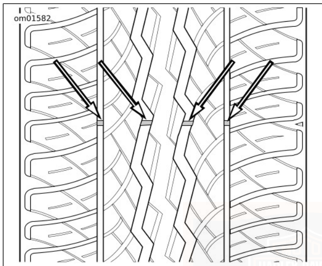
Afbeelding 62. Uiterlijk van de Dunlop-bandslijtage-indicator achter
