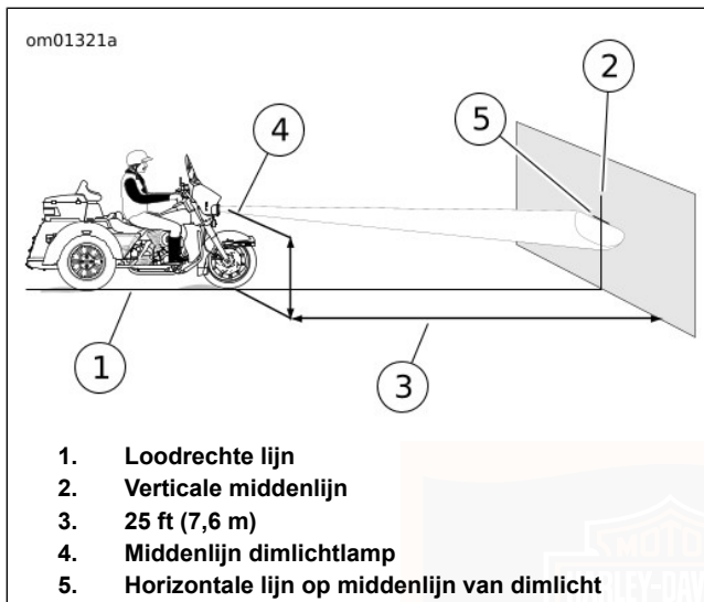
Afbeelding 65. Koplampuitlijning: LED
