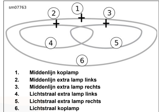
Afbeelding 67. Lampen goed afstellen: LED-lamp KOPLAMPUITLIJNING: HDI
