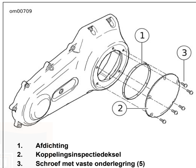
Afbeelding 46. Koppelingsdekseel
