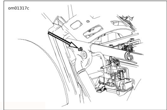
Afbeelding 24. Achterluchtveringklep
