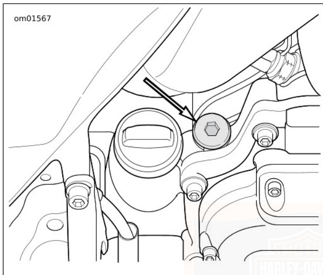
Afbeelding 42. Locatie van versnellingsbakpeilstok
