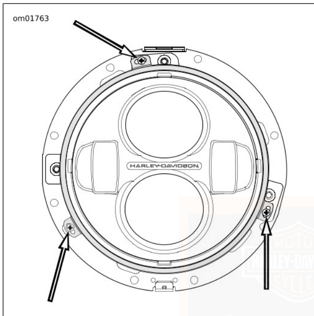
Afbeelding 64. Sluitbouten van koplamp
