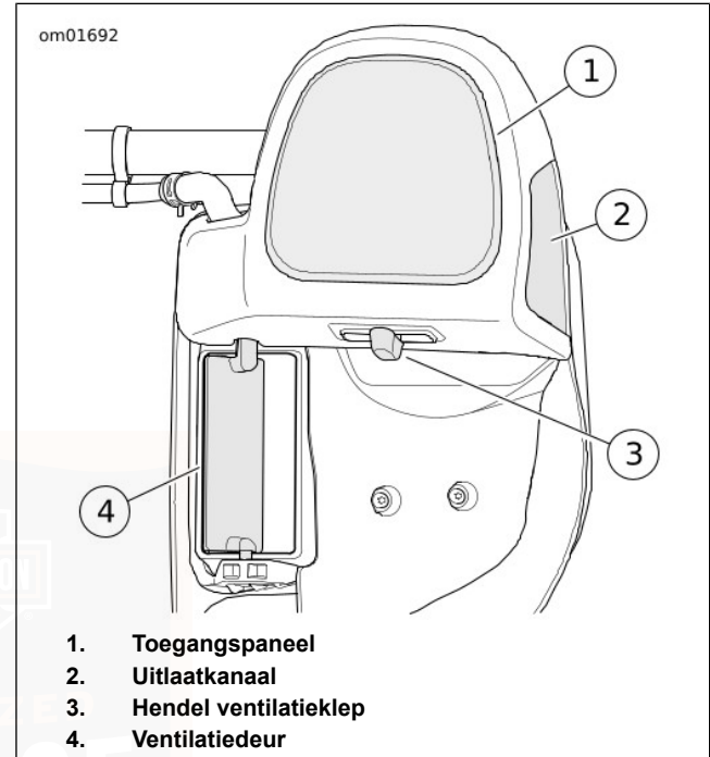
Afbeelding 32. Onderkuipen: Twin-Cooled-motorfietsen
