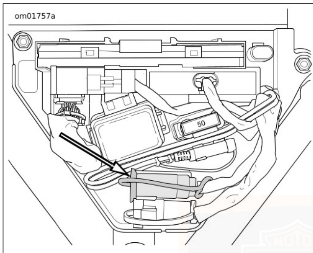
Afbeelding 11. Accessoirecontact (onder linkerzijafdekking)
