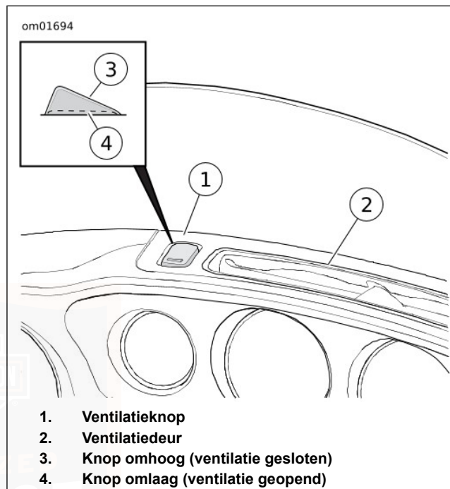
Afbeelding 30. Splitstream-ventilatie kuip AFSTELBARE WINDGELEIDERS
