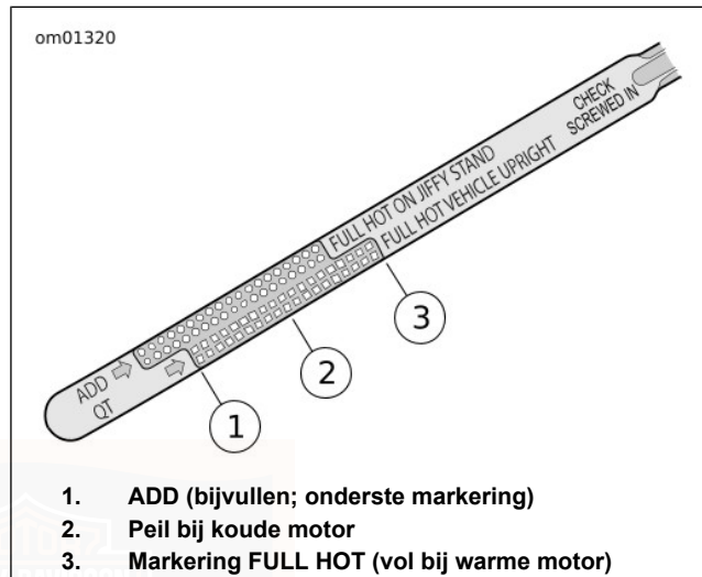
Afbeelding 39. Oliepeilstok (schaal VEHICLE UPRIGHT [voertuig staat rechtop])
