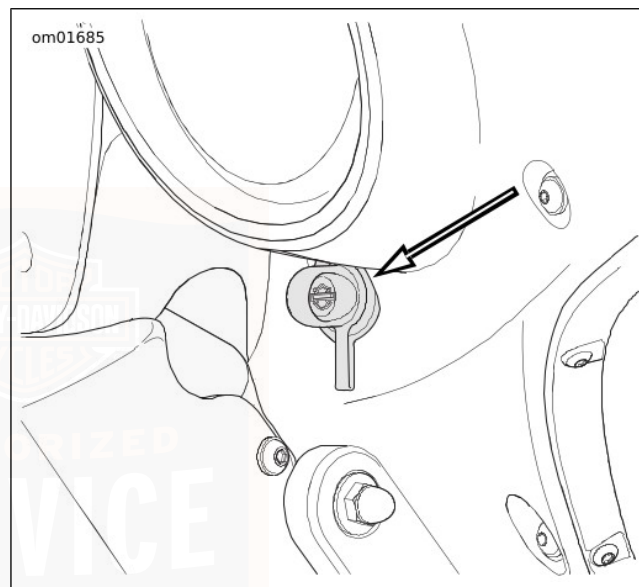
Afbeelding 29. Voedingsaansluiting op kuip
