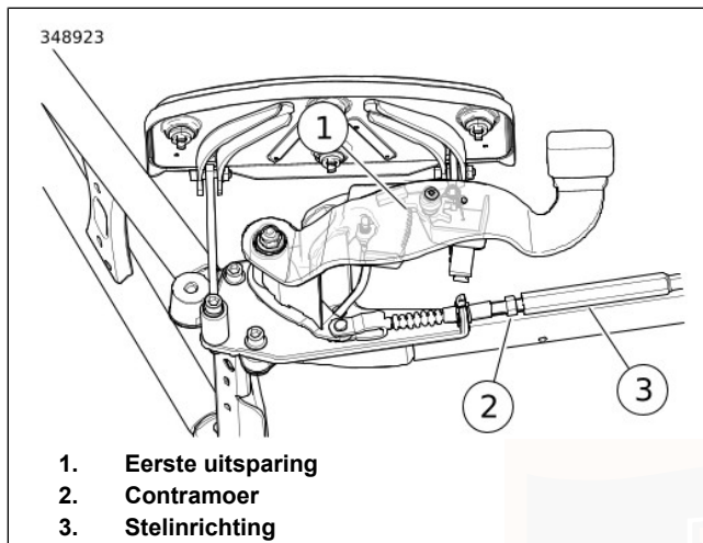
Afbeelding 56. Afstellen parkeerrem
