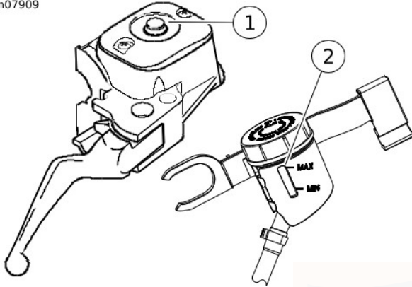
Afbeelding 53. Kijkglas remvloeistof (standaard)
