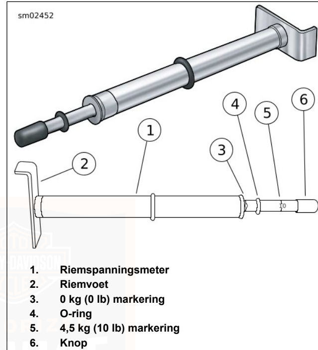
Afbeelding 49. Riemsanningsmeter
