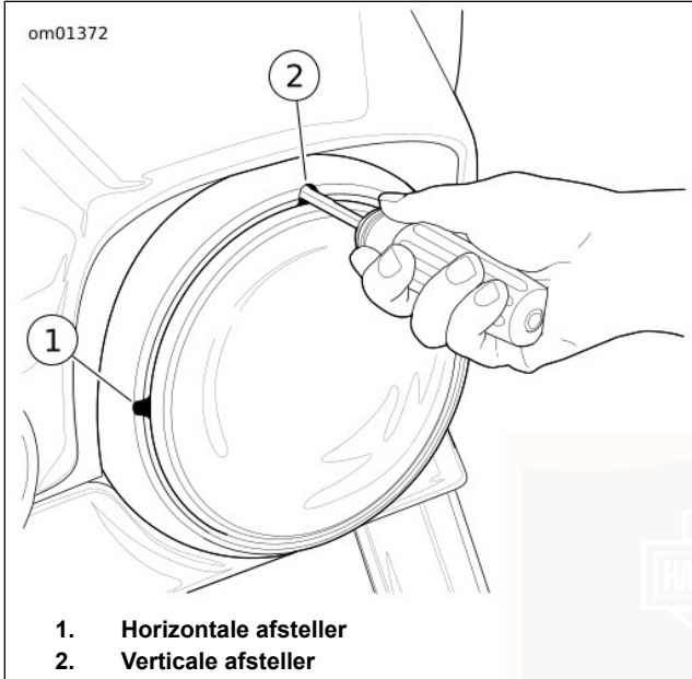
Afbeelding 66. Afstelling van de koplamp (standaard)
