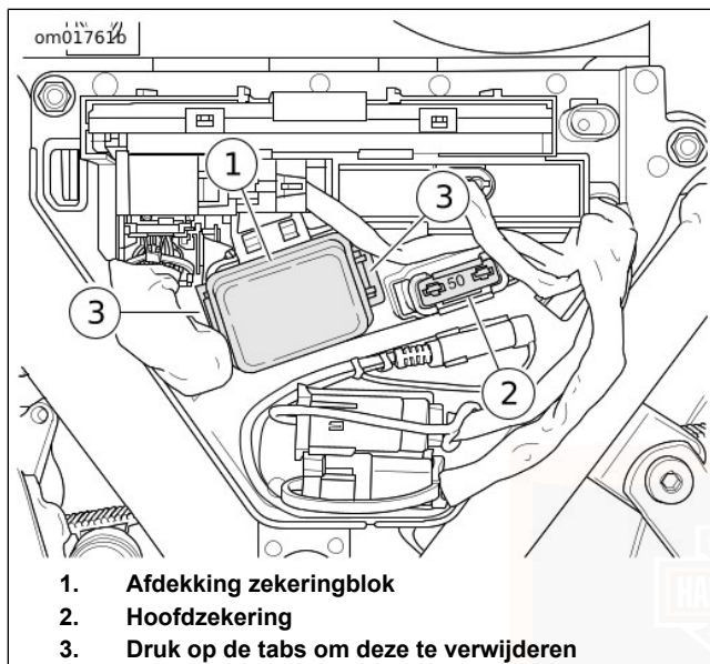
Afbeelding 82. Zekeringblokken (onder linkerzijafdekking)
