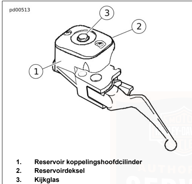
Afbeelding 52. Reservoir koppelingshoofdcilinder
