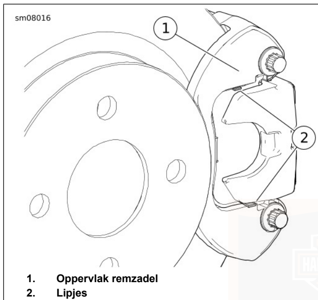
Afbeelding 55. Inspecteren van de achterremblokken
