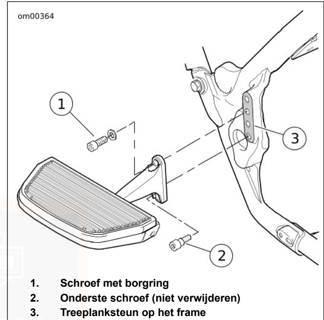
Afbeelding 21. Passagierstreeplank
