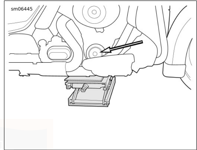
Afbeelding 57. Krikpositie voorzijde
