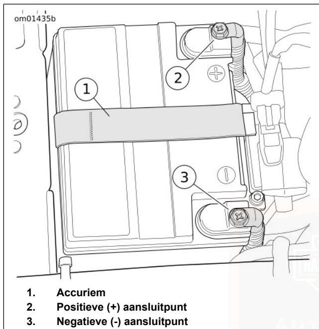
Afbeelding 79. Accuruimte
