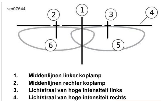
Afbeelding 69. Koplampuitlijning: HDI
