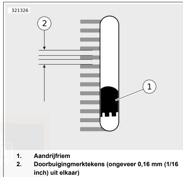
Afbeelding 51. Riemdoorbuigingsvenster
