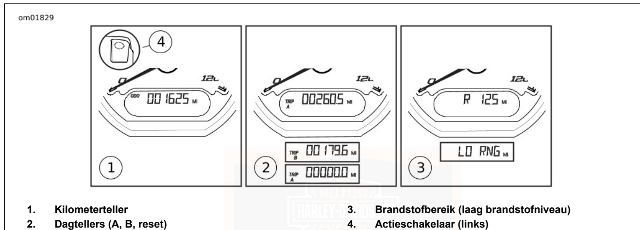
Afbeelding 6. Kilometertellerfuncties
