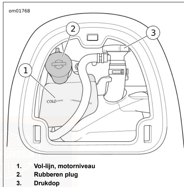
Afbeelding 48. Koelvloeistofpeil
