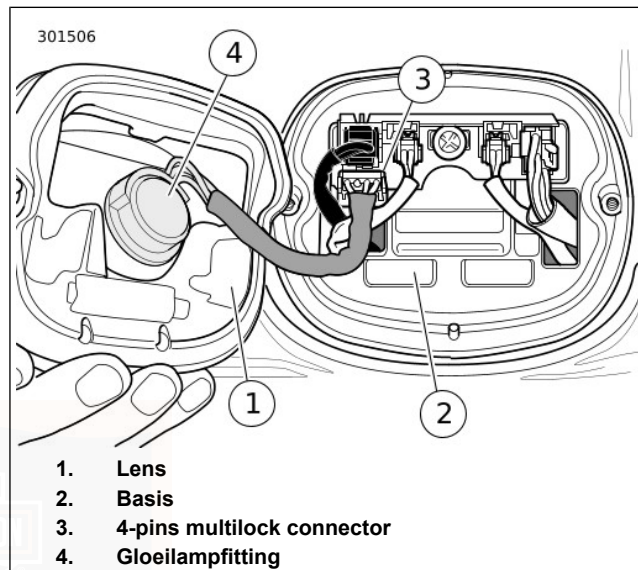
Afbeelding 72. Achterlicht
