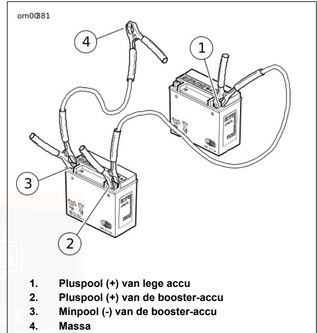
Afbeelding 80. Aansluitingen van hulpstartkabels
