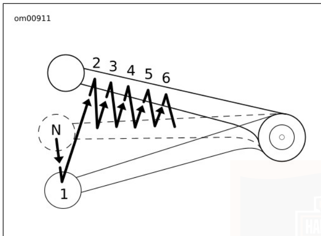
Afbeelding 36. Schakelvolgorde: Opschakelen
