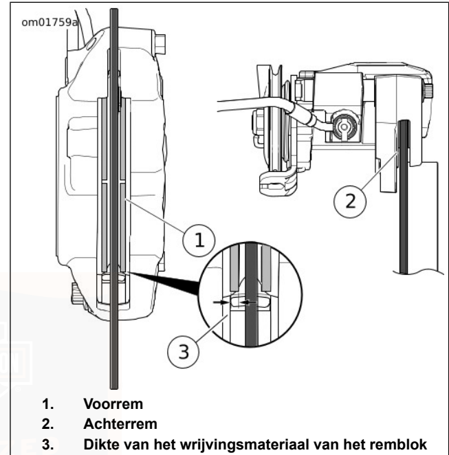
Afbeelding 54. Remwrijvingsmateriaal
