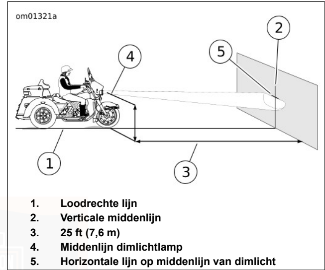
Afbeelding 68. Koplampuitlijning: LED
