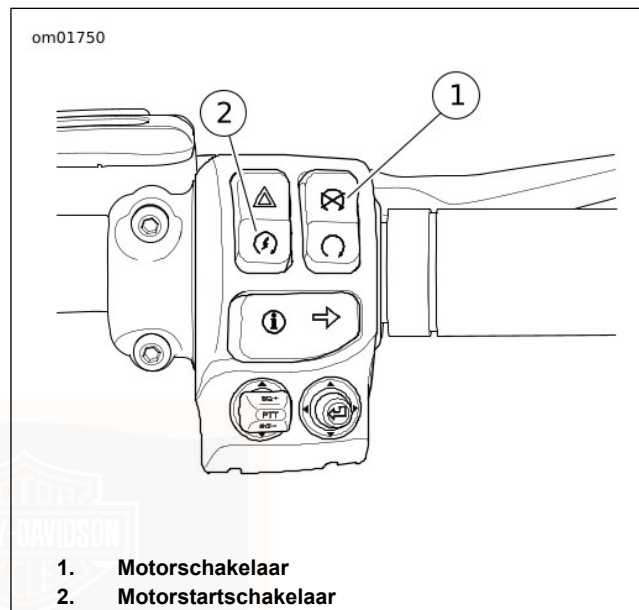
Afbeelding 35. Bedieningselementen op rechter stuurhelft
