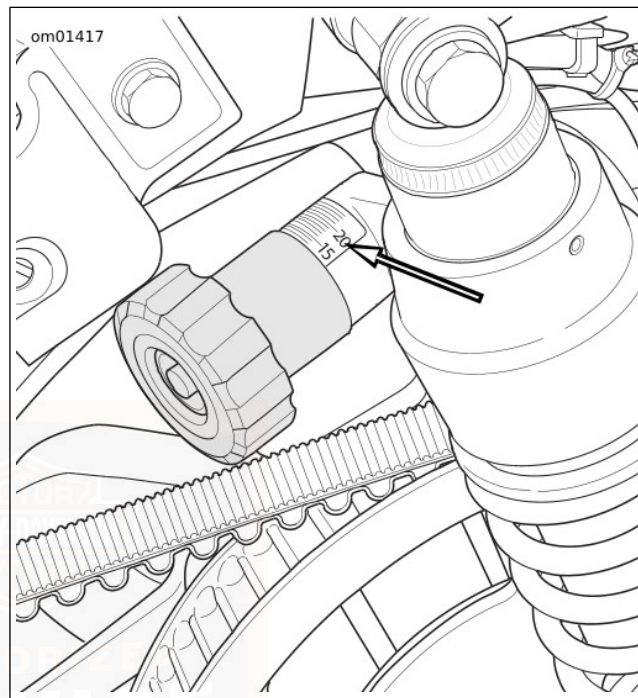
Afbeelding 12. Voorbelastingsafstellingknop
