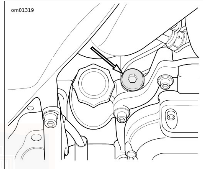
Afbeelding 63. Locatie van versnellingsbakvuldop/-peilstok
