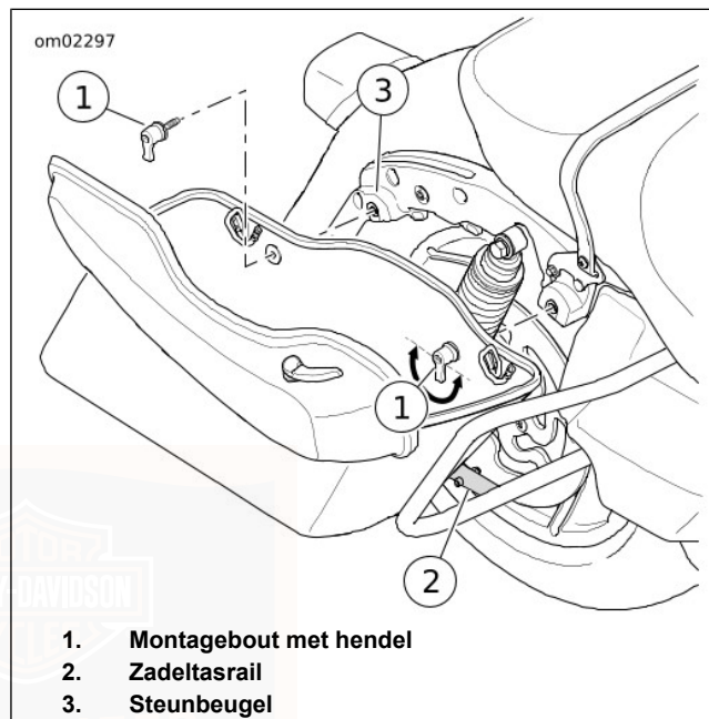
Afbeelding 52. Verwijderen/bevestigen van de zadeltas
