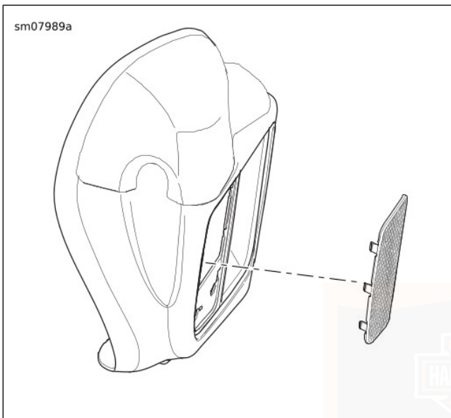
Afbeelding 73. Grillepaneel onderkuip
