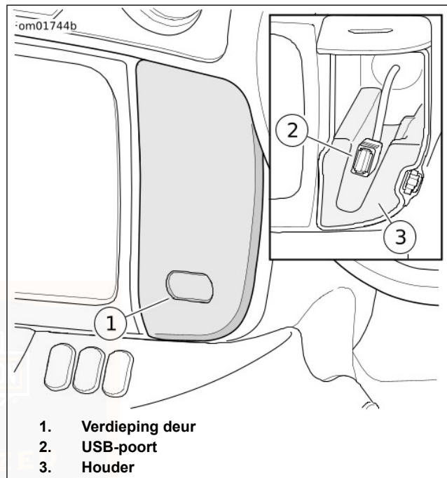
Afbeelding 36. Mediacompartiment VOEDINGSAANSLUITING
