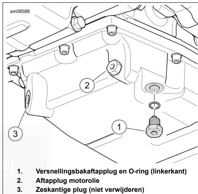
Afbeelding 65. Versnellingsbakaftap
