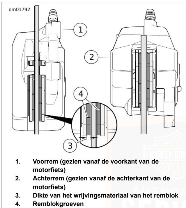
Afbeelding 71. Wrijvingsmateriaal van het remblok
