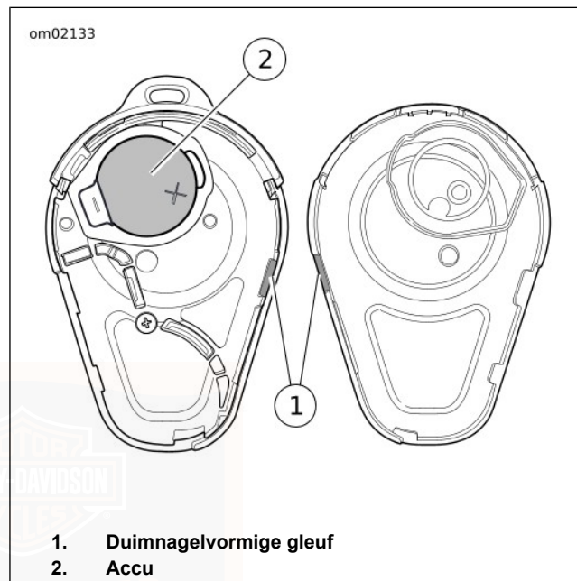
Afbeelding 15. Afstandsbedieningsbatterij
