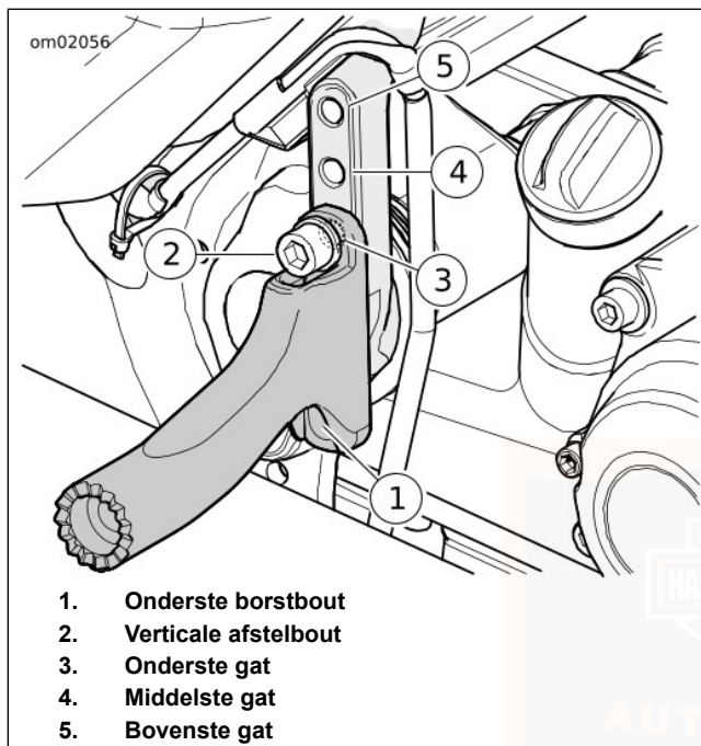
Afbeelding 44. Hoogte-afstelling treeplank (draaiende arm en treeplank verwijderd)
