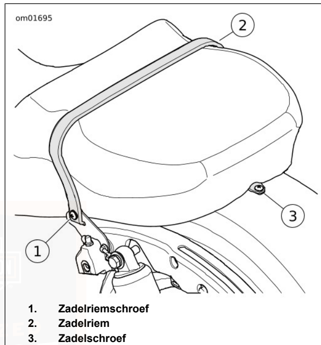
Afbeelding 95. Zadelriemschroef
