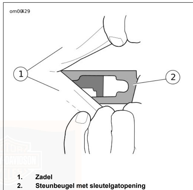
Afbeelding 47. Montagesteun bestuurdersrugsteun KUIPVENTILATIE-OPENINGEN
