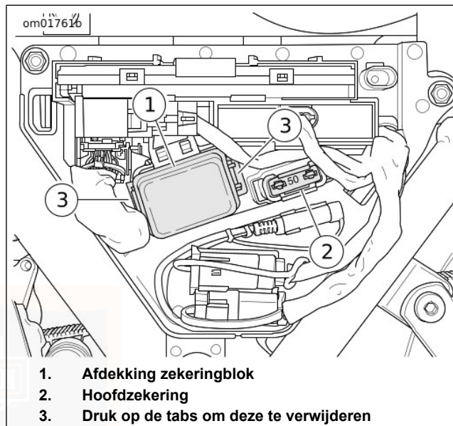
Afbeelding 86. Zekeringblokken (onder linkerzijafdekking)
