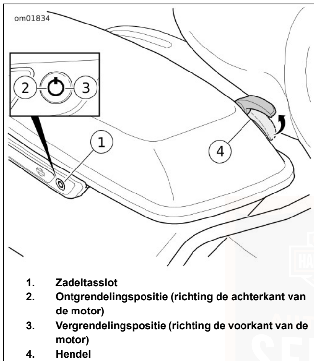
Afbeelding 51. Zadeltas
