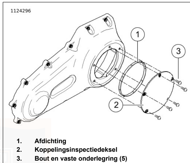
Afbeelding 68. Koppelingsdeksel (standaard)
