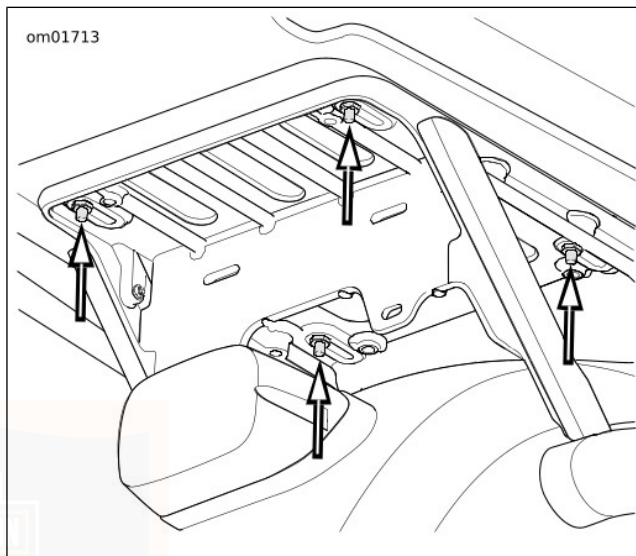
Afbeelding 55. Positie Tour-Pak afstellen
