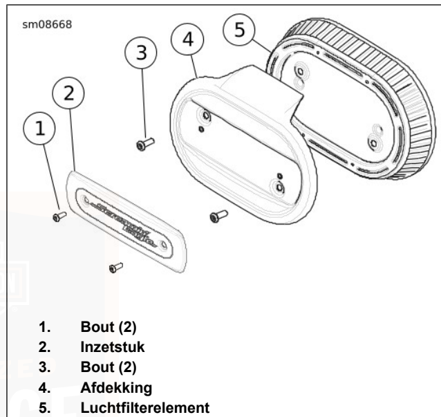
Afbeelding 77. Luchtfilterelement
