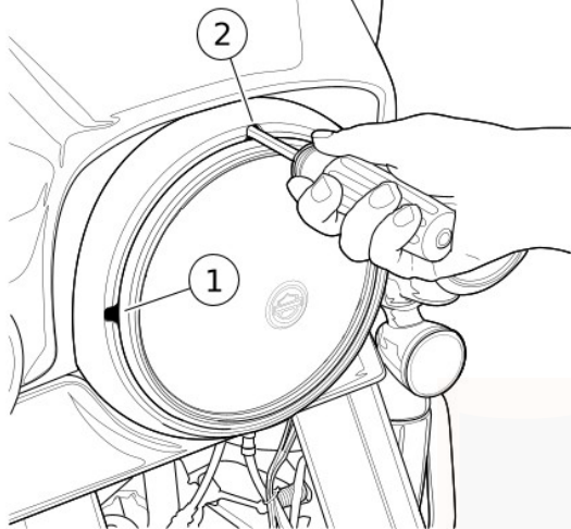
Afbeelding 90. Koplampstelschroeven: Alle kuipen, behalve op het frame gemonteerde kuip (typisch)
