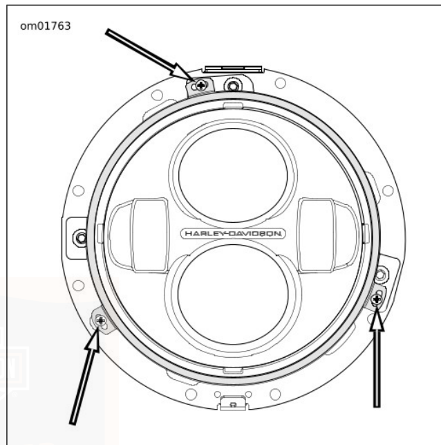
Afbeelding 91. Sluitbouten van koplamp STEL EXTRA-/MISTLAMPEN AF
