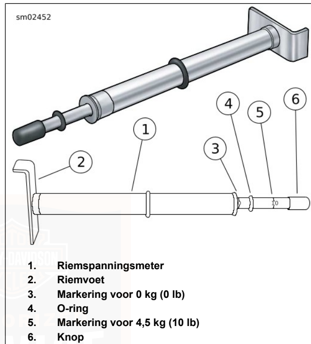
Afbeelding 74. Riemspanningsmeter
