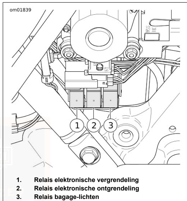
Afbeelding 88. Relais elektronische vergrendeling (onder rechterzijafdekking)
