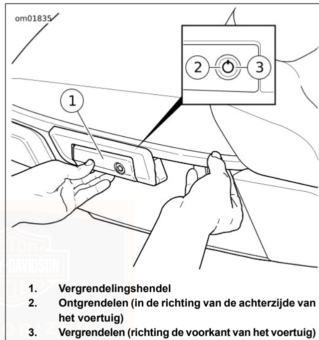
Afbeelding 54. Tour-Pak
