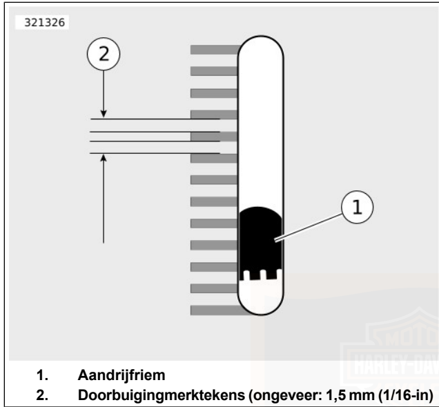
Afbeelding 75. Riemdoorbuigingsvenster
