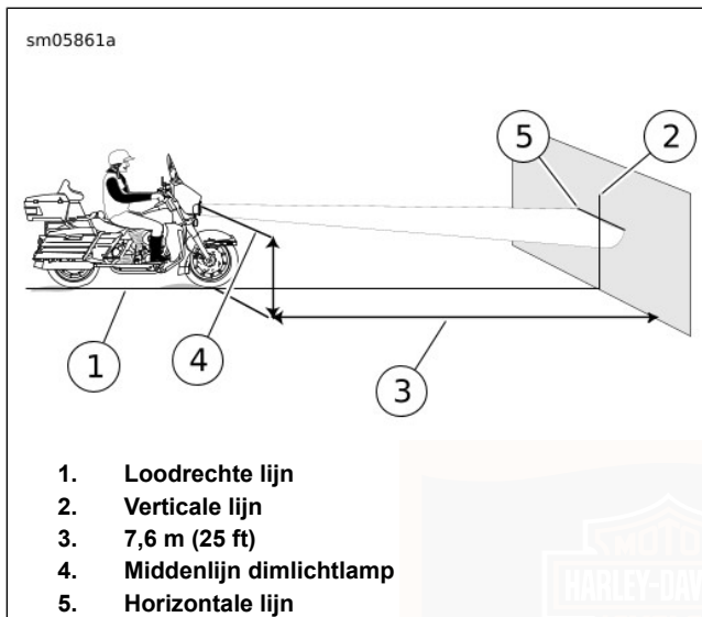
Afbeelding 89. Koplampuitlijning: LED (standaard)
