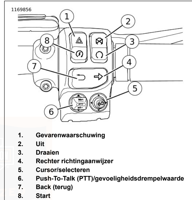
Afbeelding 39. Rechter stuurschakelaarmodule
