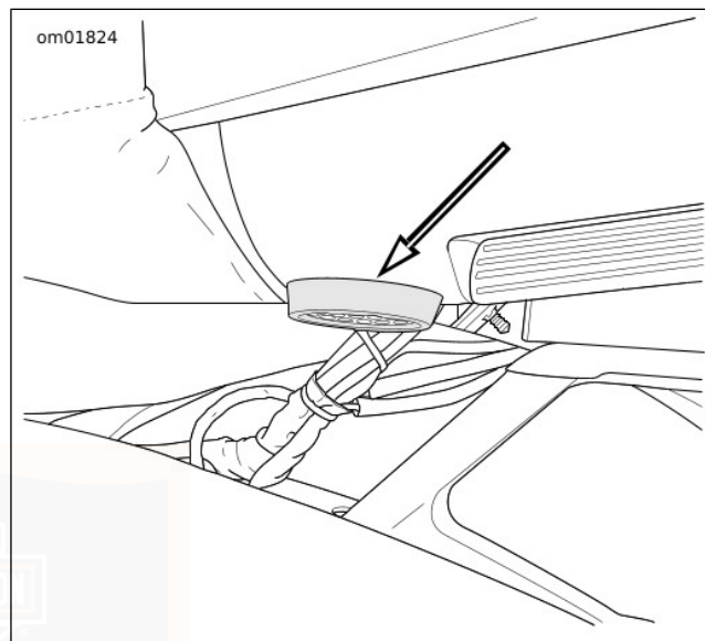
Afbeelding 58. Zadeltaslicht (onder Tour-Pak)
