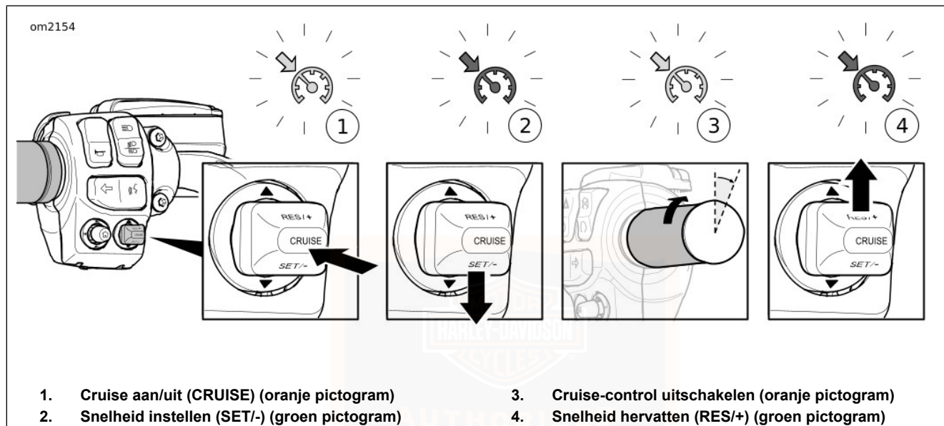
Afbeelding 23. Cruise-control (typisch)
