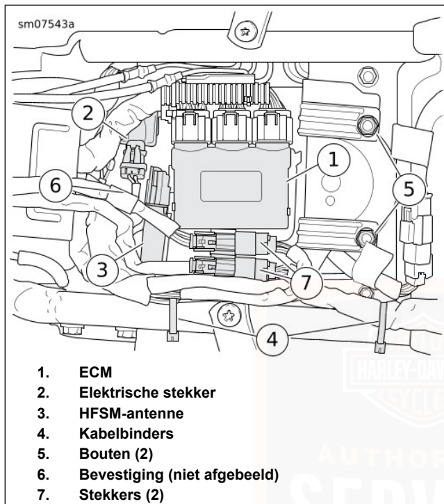
Afbeelding 84. Bovenste accuhouder
