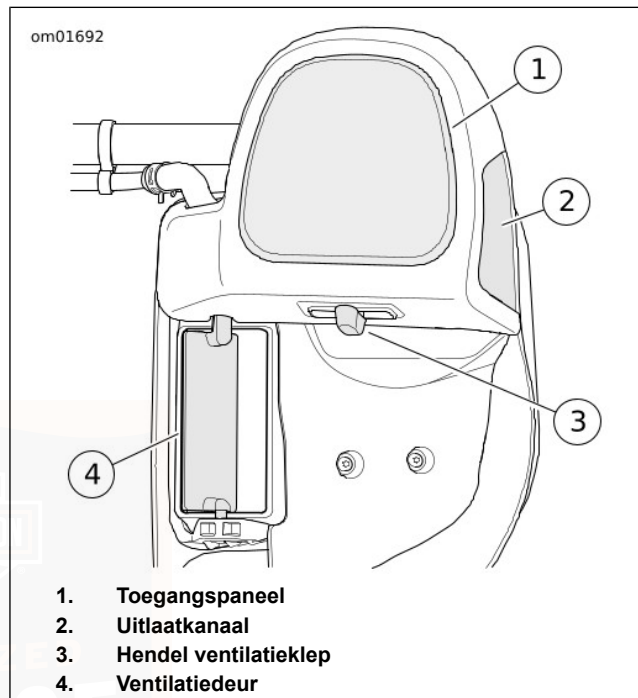
Afbeelding 50. Onderkuipen: Twin-Cooled-modellen
