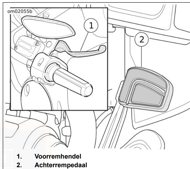
Afbeelding 40. Rembediening
