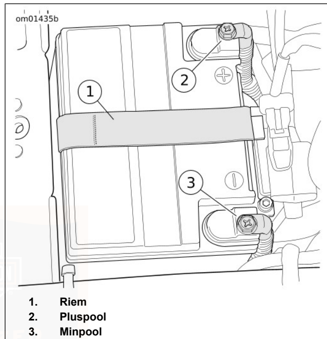
Afbeelding 85. Accuimte
