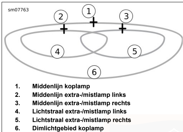
Afbeelding 92. Koplamppatroon: LED-uitvoering met extra-/mistlampen
