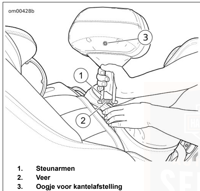
Afbeelding 46. Installeren van bestuurdersrugsteun
