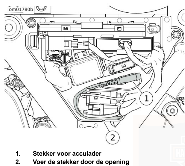
Afbeelding 82. Stekker acculader (onder linkerzijafdekking)
