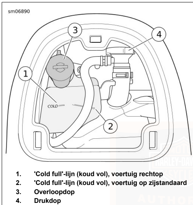
Afbeelding 72. Koelvloeistofpeil
