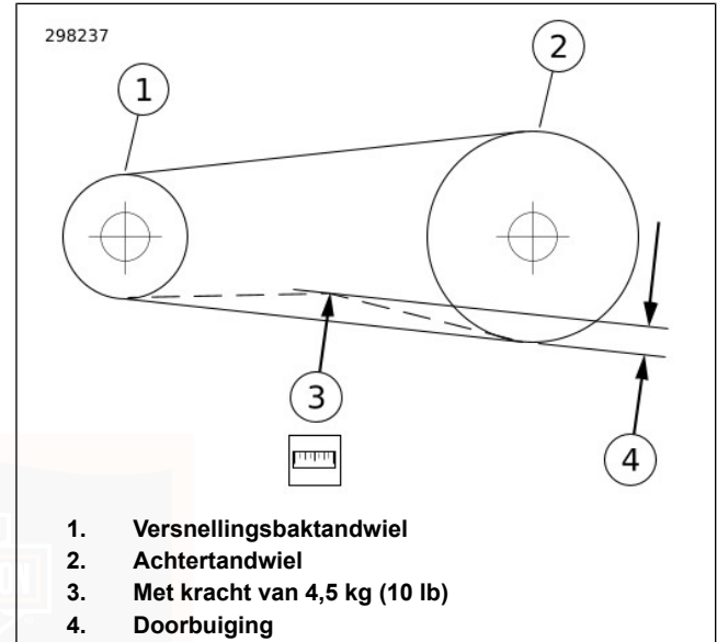
Afbeelding 76. Doorbuiging van riem controleren
