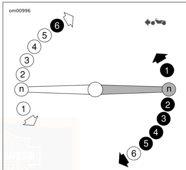
Afbeelding 10. Hak-teen-schakelpedaal ANTIBLOKKEERSYSTEEM (ABS)
