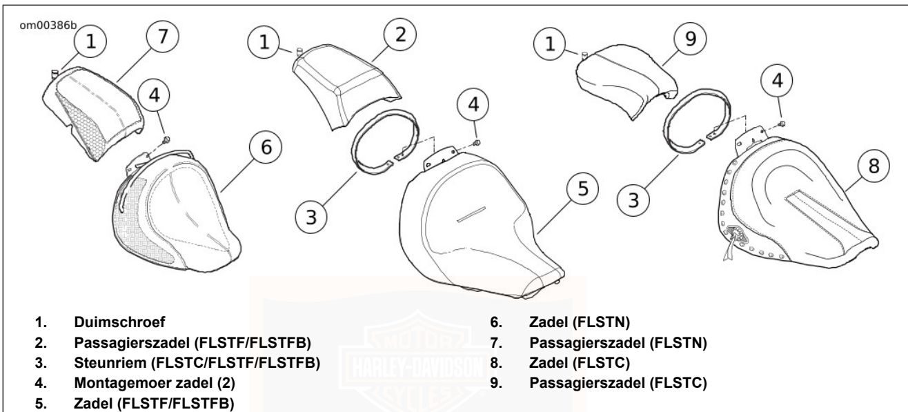
Afbeelding 57. Zadel: FLSTN/C/F/FB-modellen
