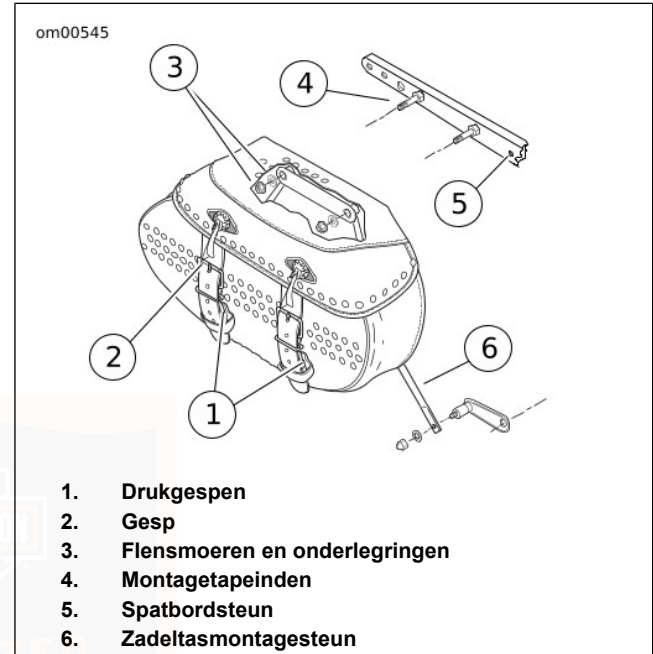
Afbeelding 15. Zadeltas: FLSTC
