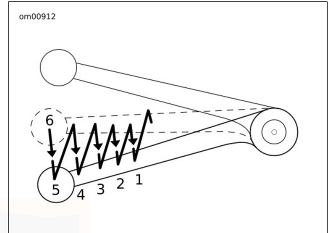
Afbeelding 24. Schakelvolgorde: Terugschakelen
