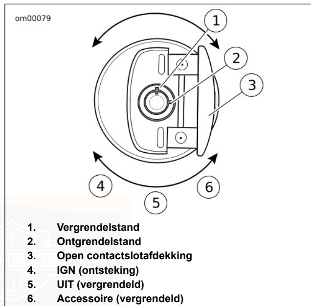
Afbeelding 4. Contactslot: Softail-modellen (behalve FXS)
