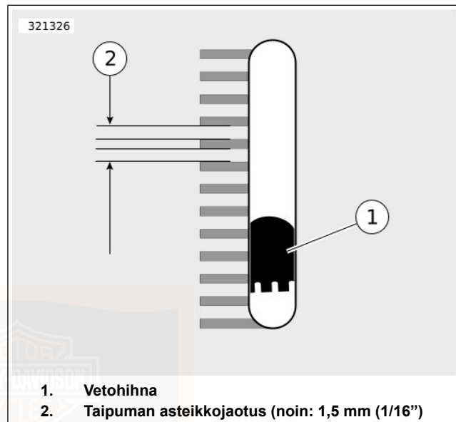
Kuva 59. Hihnan taipuman tarkistusikkuna
