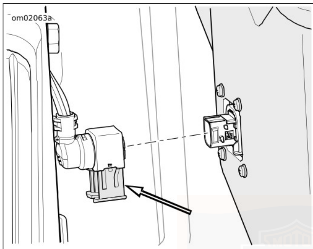
Kuva 43. Oikean liittimen lukitustanko
