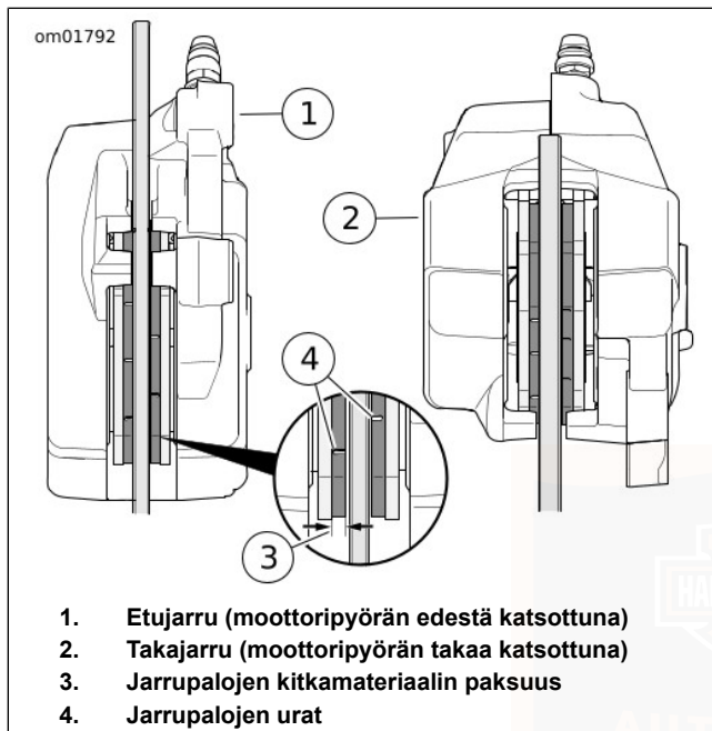
Kuva 57. Jarrupalojen kitkamateriaali
