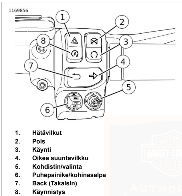
Kuva 20. Oikea kytkinmoduuli
