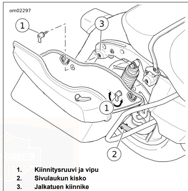
Kuva 42. Sivulaukun irrotus/asennus
