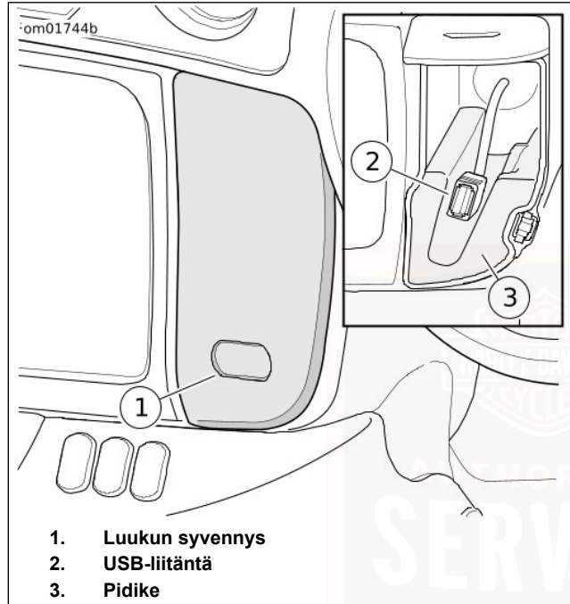
Kuva 32. Medialokero
