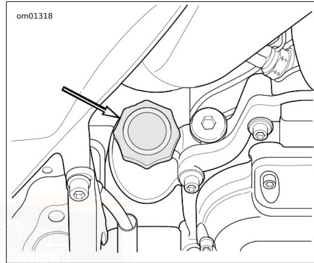
Kuva 45. Moottoriöljyn täyttötulppa
