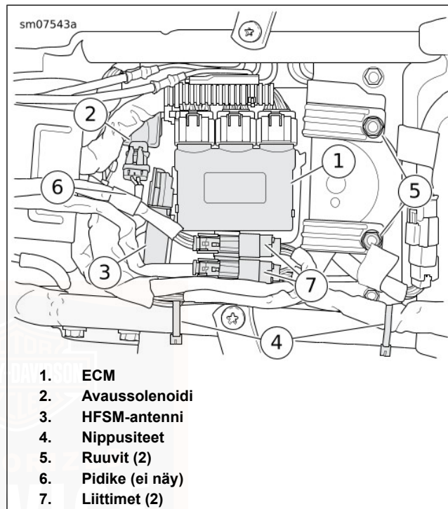
Kuva 68. Yläteline
