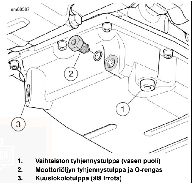
Kuva 47. Öljypohja
