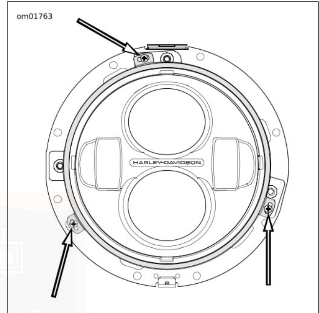
Kuva 75. Ajovalon pidikeruuvit
