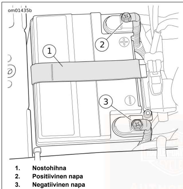
Kuva 69. Akukulokero
