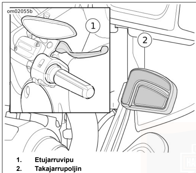
Kuva 35. Jarrujen hallintalaitteet
