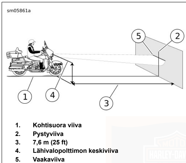
Kuva 73. Ajovalon kohdistaminen: LED-tyyppi (tyypillinen)
