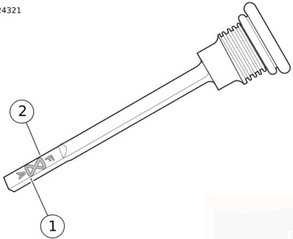
Kuva 50. Vaihteistoöljyn taso
