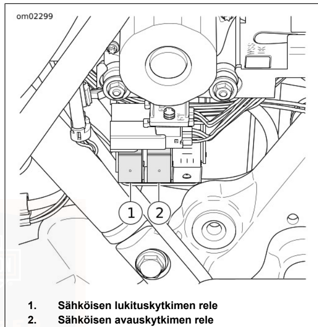
Kuva 72. Sähkölukkojen releet (oikean sivukatteen alla)
