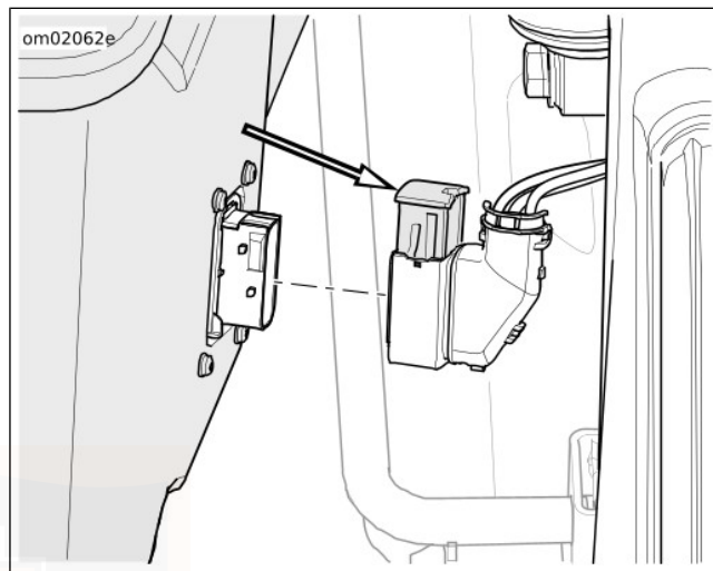
Kuva 44. Vasemman liittimen lukitustanko
