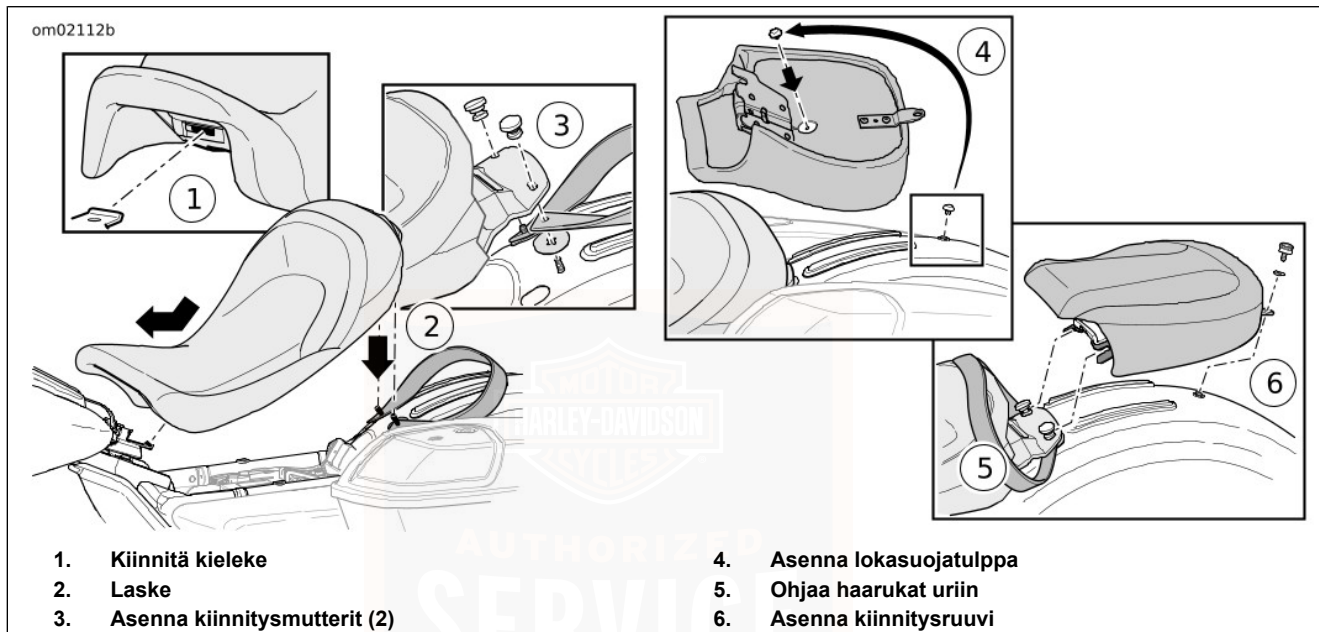
Kuva 76. Etu- ja takasatulan asentaminen
