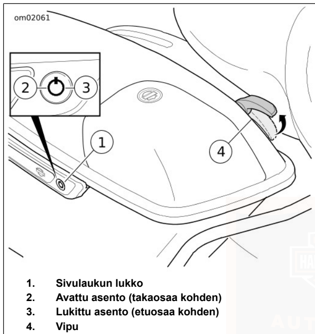
Kuva 41. Sivulaukku
