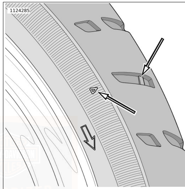
Kuva 63. Renkaan kulumisilmaisimen paikan ilmaisin
