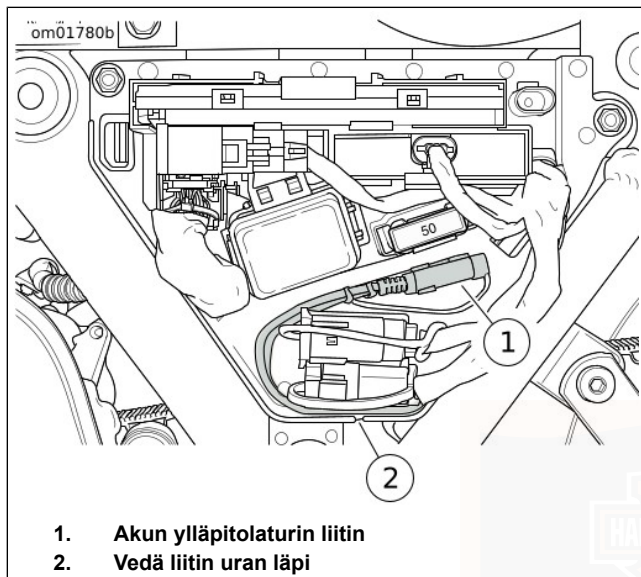
Kuva 66. Akun ylläpitolaturin liitin (vasemman sivukatteen alla)
