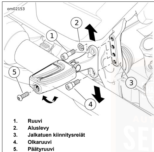
Kuva 39. Matkustajan jalkatuki
