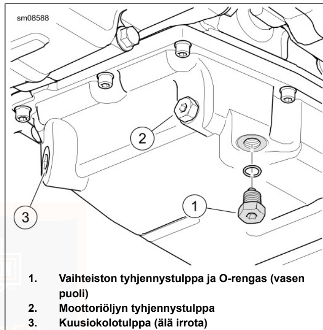
Kuva 51. Vaihteiston tyhjennys
