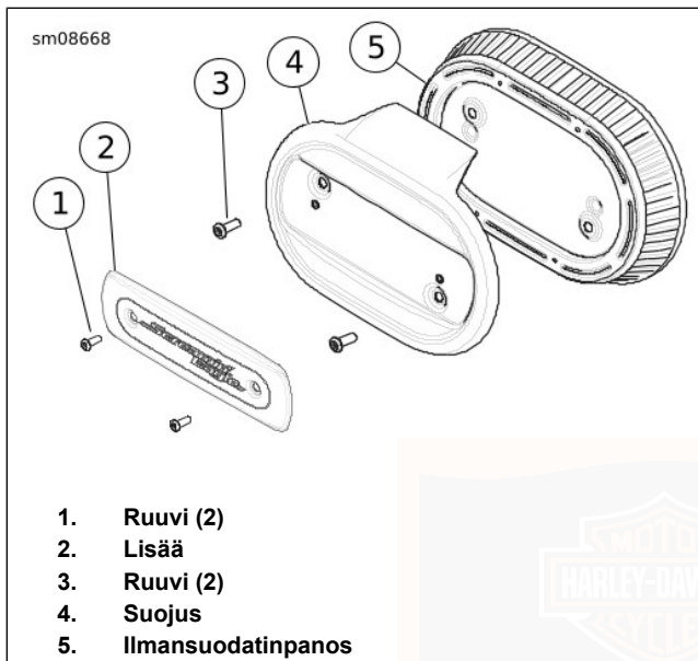
Kuva 61. Ilmansuodatin
