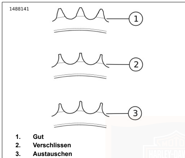
Abbildung 61. Zahnradzahnzustand
