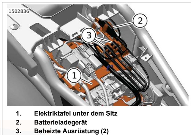
Abbildung 66. Unter dem Sitz
