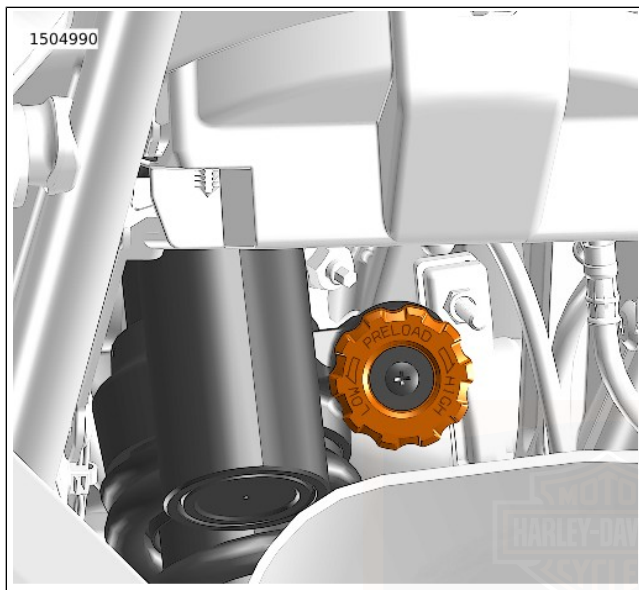
Abbildung 17. Vorspannungseinsteller
