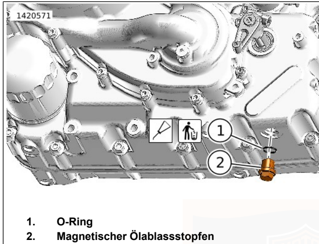
Abbildung 54. Ölablassschraube
