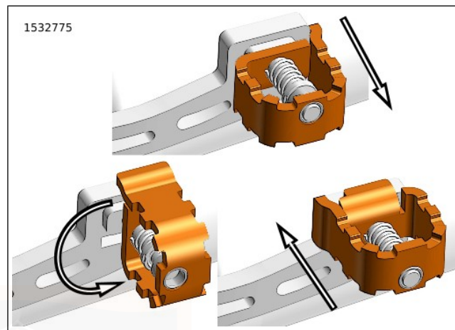
Abbildung 46. Änderung der Bremspedalhöhe
