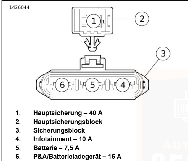
Abbildung 85. Sicherungsblöcke und Buchsenkontakte
