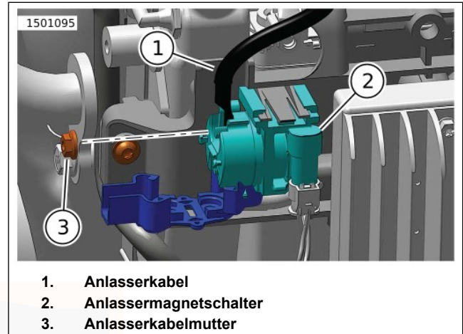
Abbildung 68. Anlasserkabel
