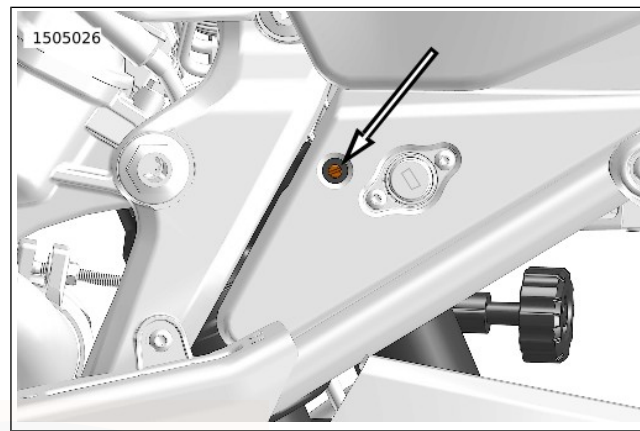
Abbildung 16. Kompressionseinsteller
