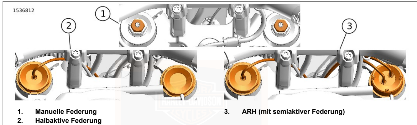
Abbildung 12. Vorderradfederungen
