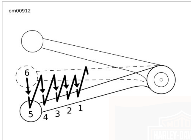
Abbildung 49. Schaltfolge: Herunterschalten WINDSCHUTZSCHEIBE
