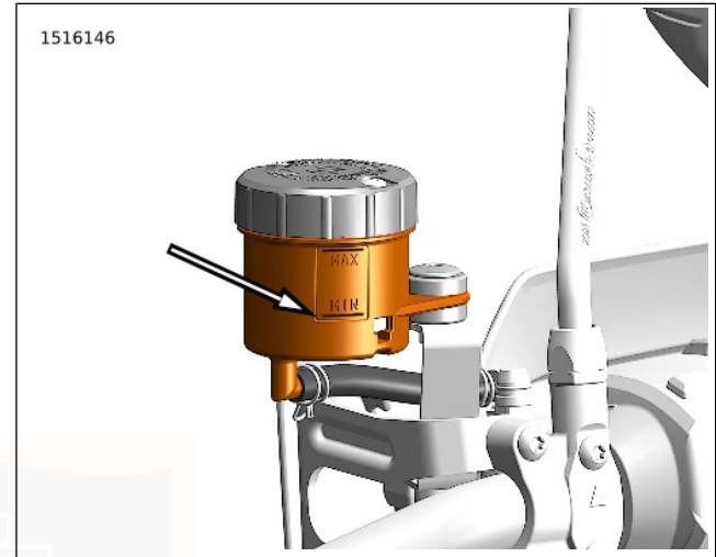
Abbildung 58. MIN-Markierung am Vorderradhauptbremszylinderbehälter
