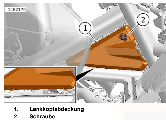
Abbildung 72. Lenkkopfabdeckung (rechte Seite abgebildet)
