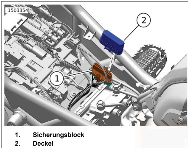
Abbildung 87. Sicherungsblock – Lage
