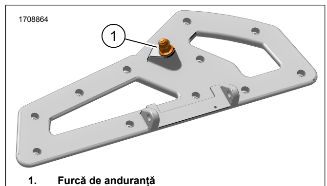
Figura 3. Suport talpă de uzură (tipic)
