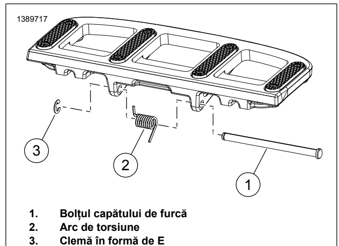
Figura 2. Kit pedală motociclist
