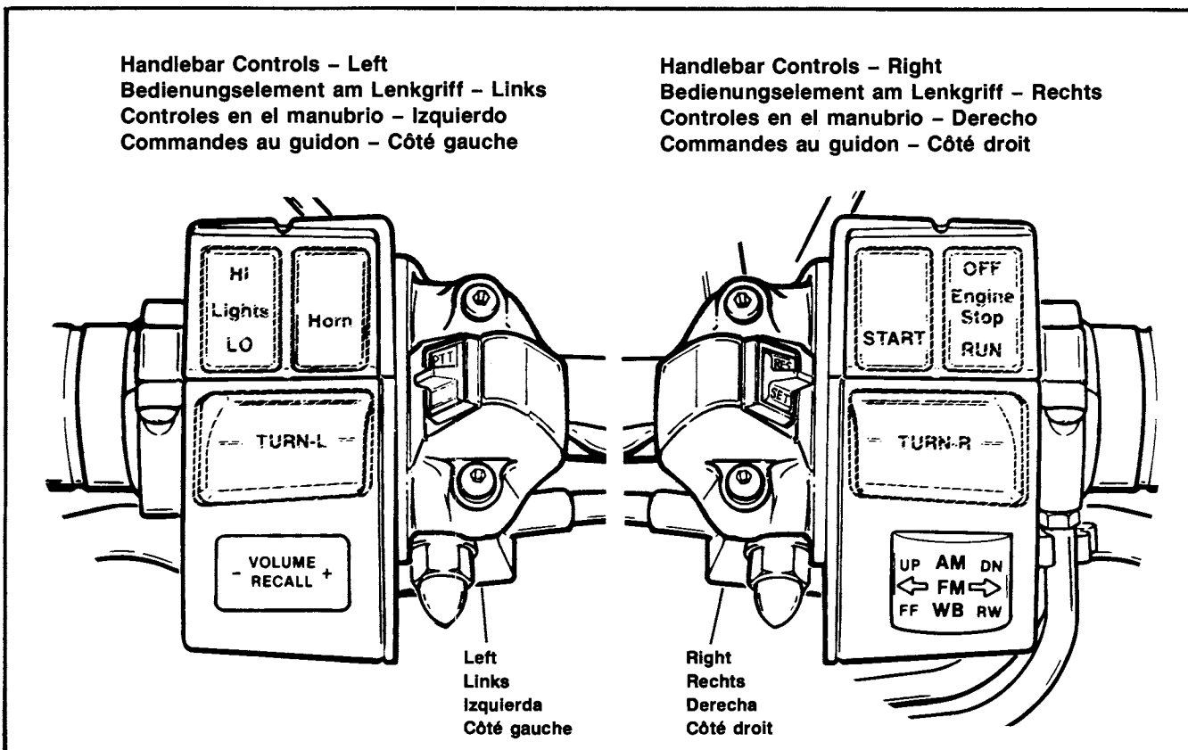
Figure 6. Commandes au guidon du système de son/régulateur de vitesse
