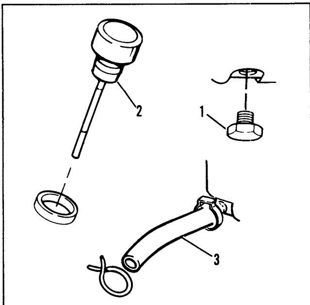
Figure 29. Vidanges réservoir huile/jauge du bouchon de remplissage
