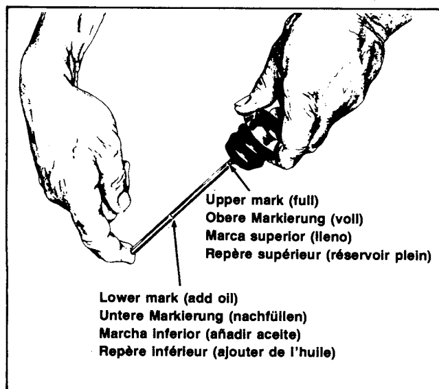
Figure 31. Jauge de niveau d'huile – modèles FXR, FLT, XLH
