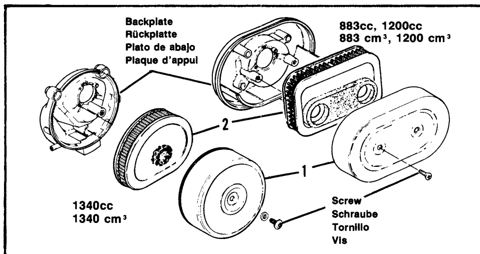
Figure 40. Air Cleaner Abbildung 40. Luftfilter Figura 40. Depurador de aire Figure 40. Filtre à air
