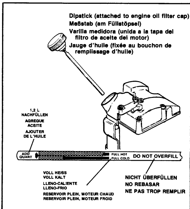
Figure 32. Bouchon de remplissage, jauge, et vidange d'huile du moteur, modèles Dyna Glide
