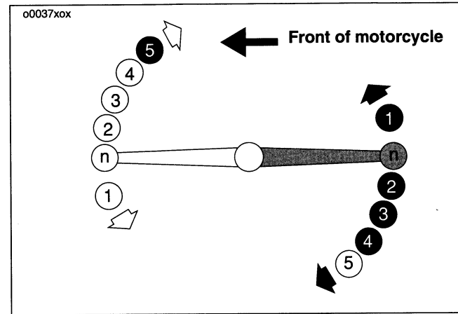
Figure 15. Heel - Toe Shift Lever
